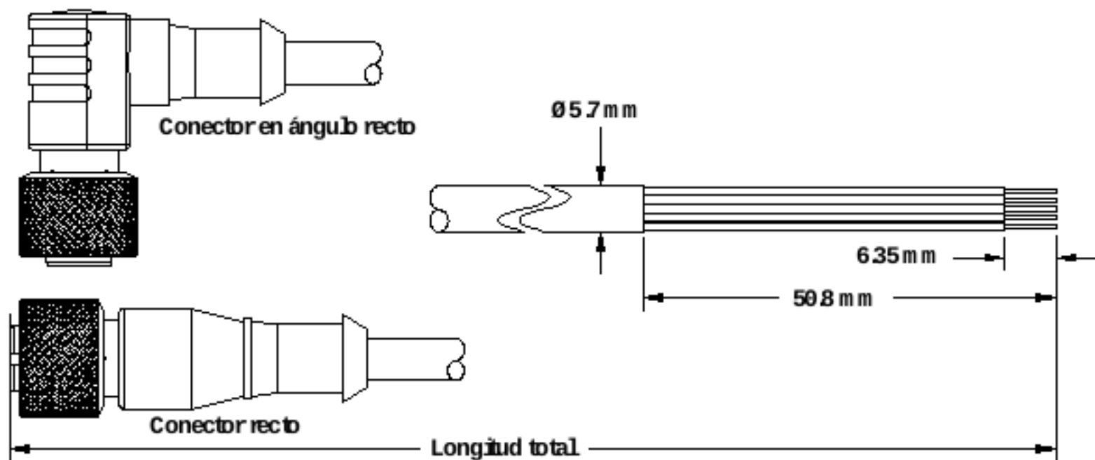
Imagen 1: Dimensiones del cable
