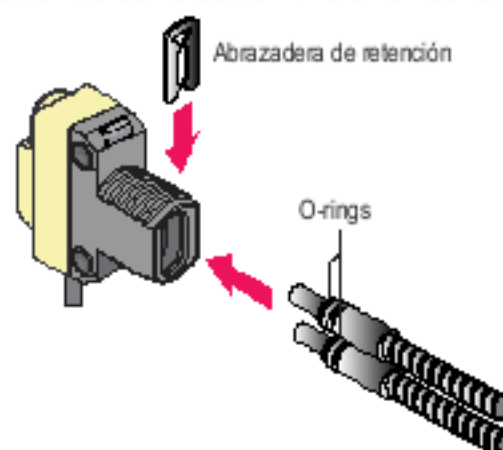
Instalación de las fibras de vidrio en un sensor QS 18
