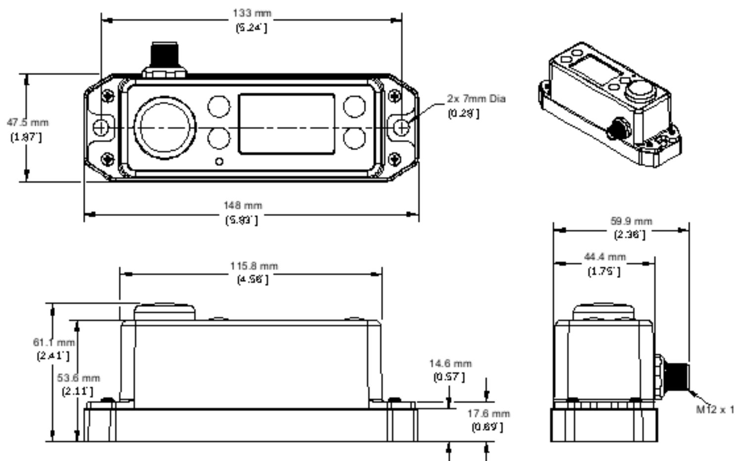
DSTS-QD dimensions
