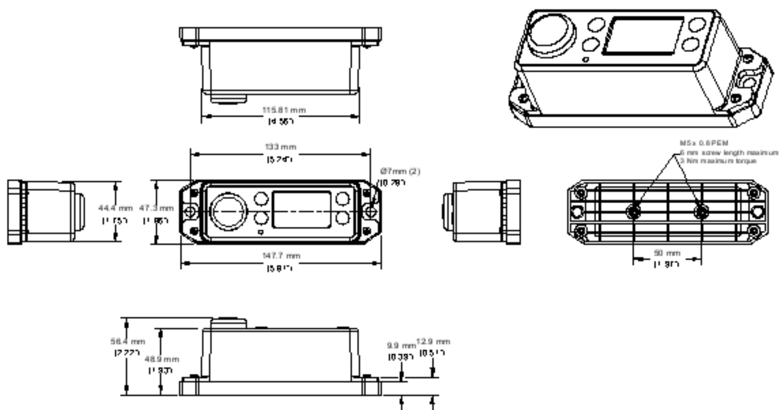
DSTS-QD dimensions
