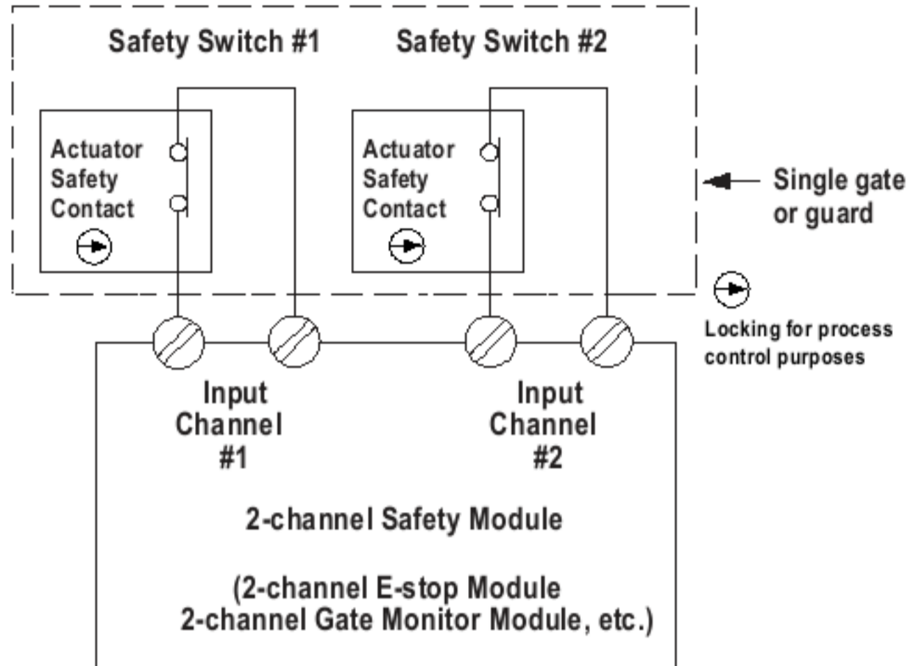
Contatti di sicurezza dell'attuatore (cerchio con il simbolo della freccia)
