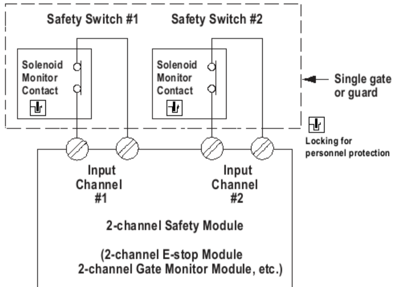
Contatti di monitoraggio solenoide (simbolo di blocco)
