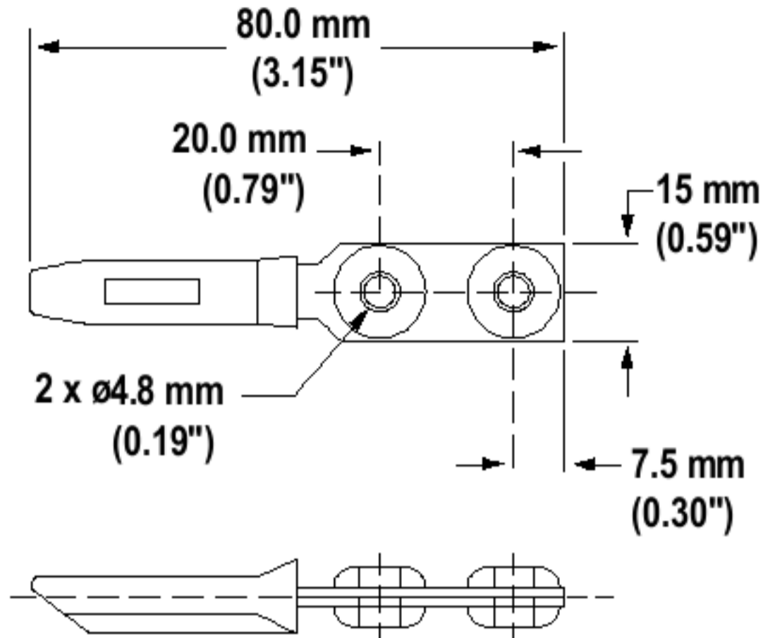
Dimensioni dell'attuatore modello SI-QM-SSA
