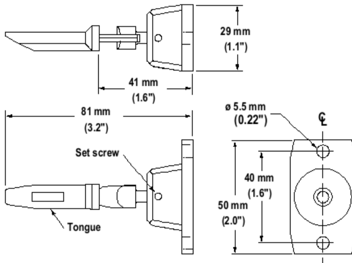
Dimensioni dell'attuatore modello SI-QM-SMFA
