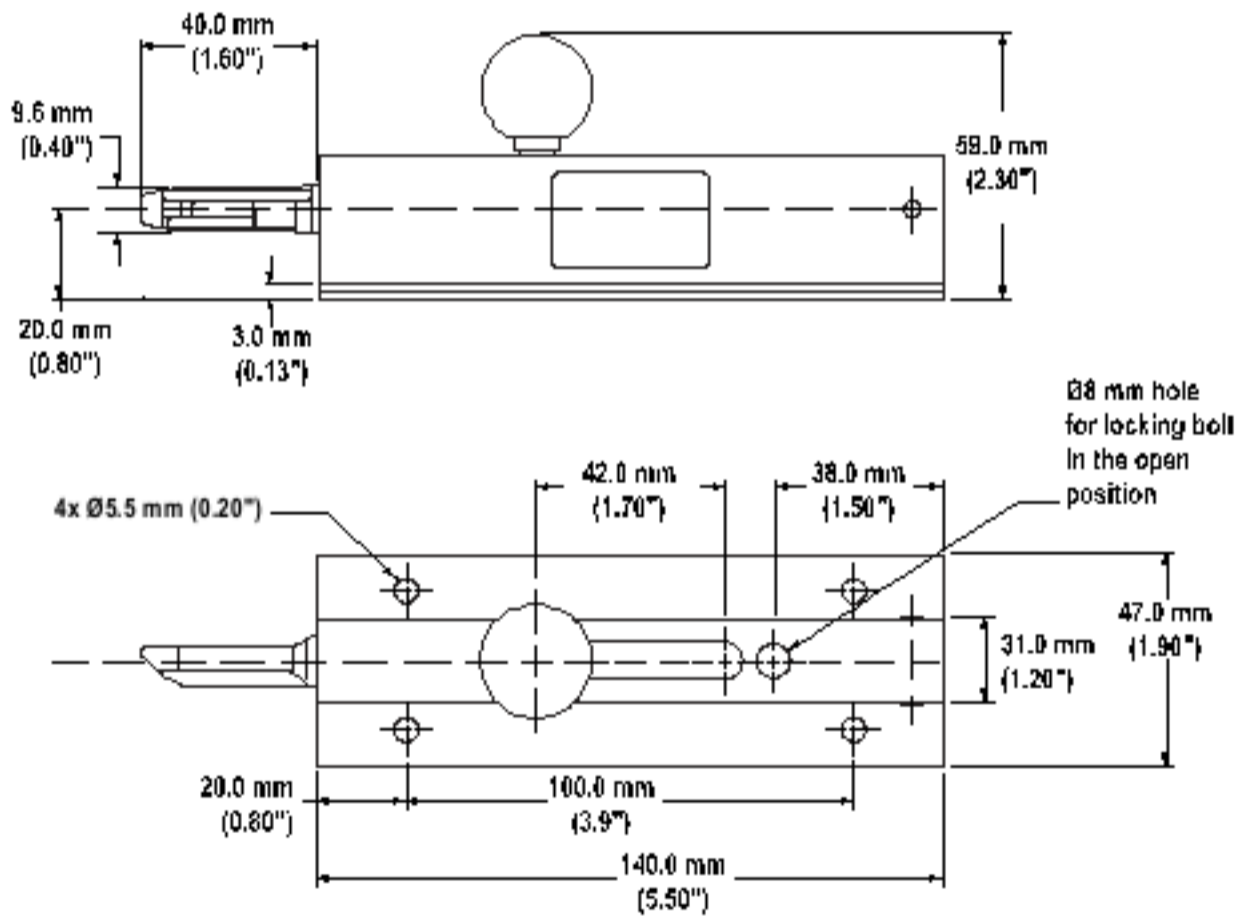
Dimensioni dell'attuatore modello SI-QM-SB
