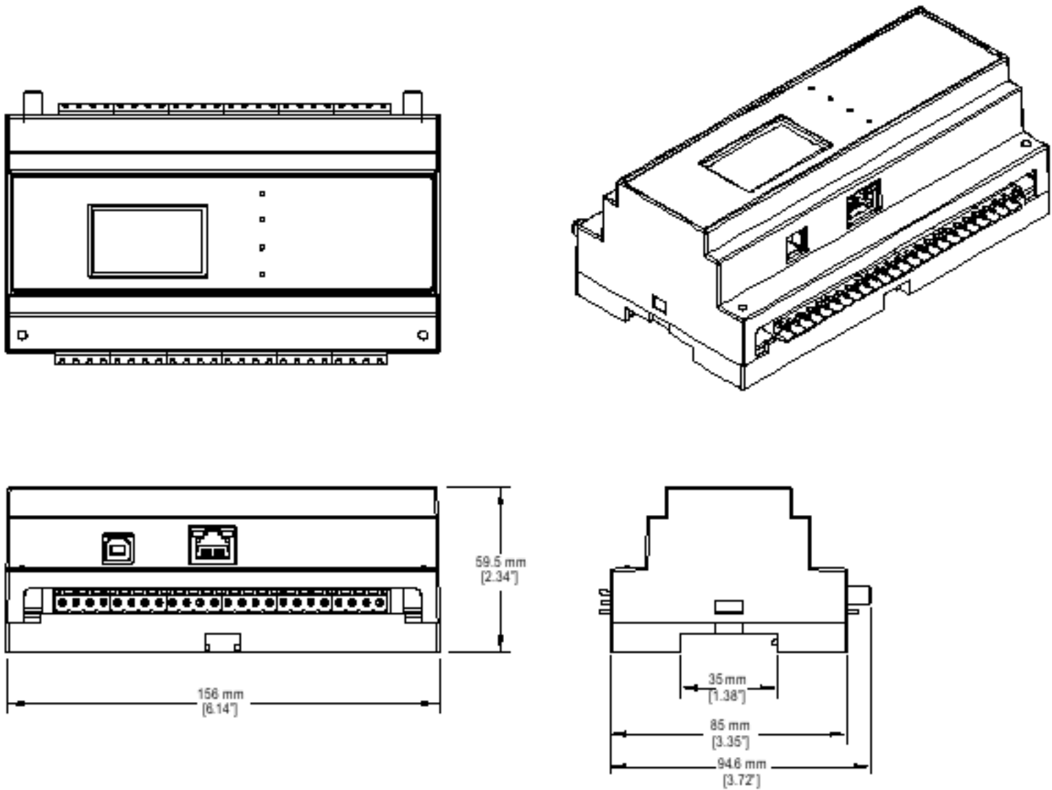
Dimensiones de los modelos DXM150 y DXM1500
