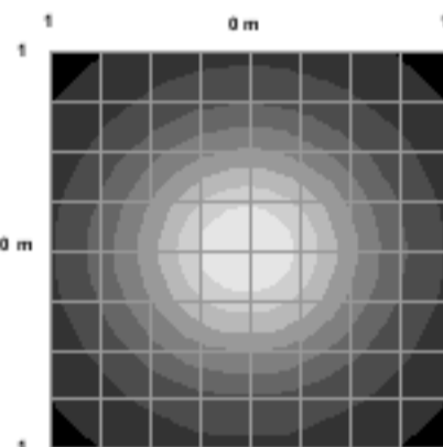
Patrón isolux
