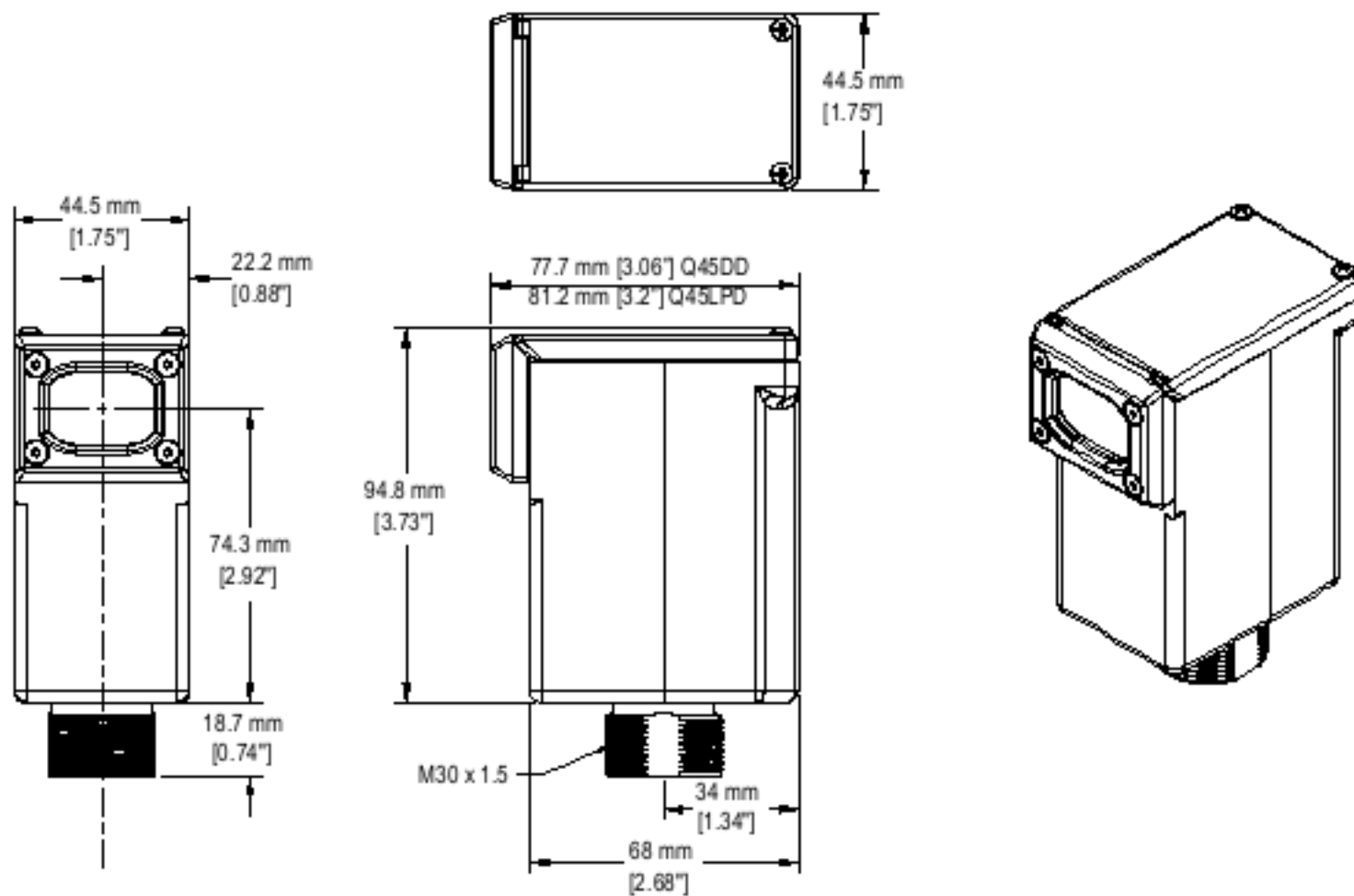
Dimensiones de los modelos Q45DD y LPD
