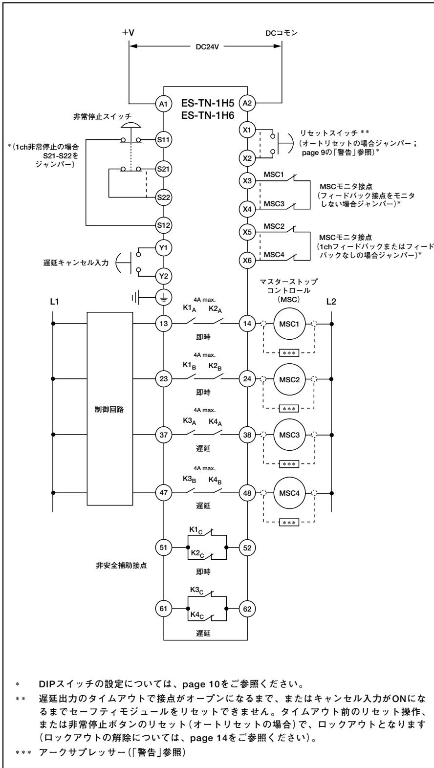
Fig.2 非常停止セーフティモジュールES-TN-1H5、-1H6の配線
