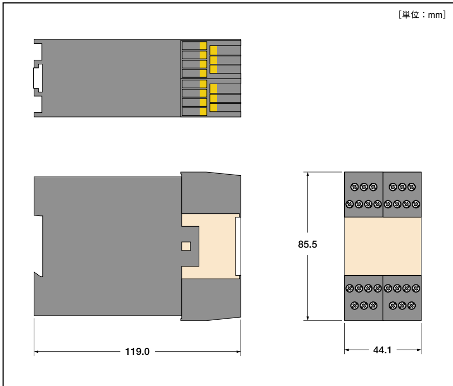
Fig.8 外形
