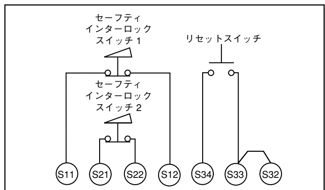
Fig.4 セーフティスイッチとマニュアルリセット使用の回路図
