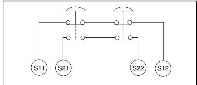
Fig.3 複数の非常停止スイッチの直列接続
