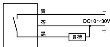
NPN出力 (ケーブルタイプ)
