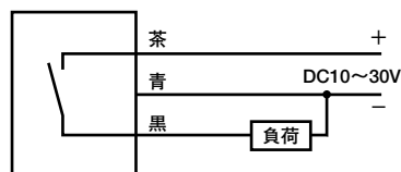
PNP出力 (ケーブルタイプ)
