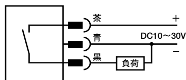
PNP出力 (コネクタタイプ)
