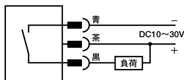
NPN出力 (コネクタタイプ)
