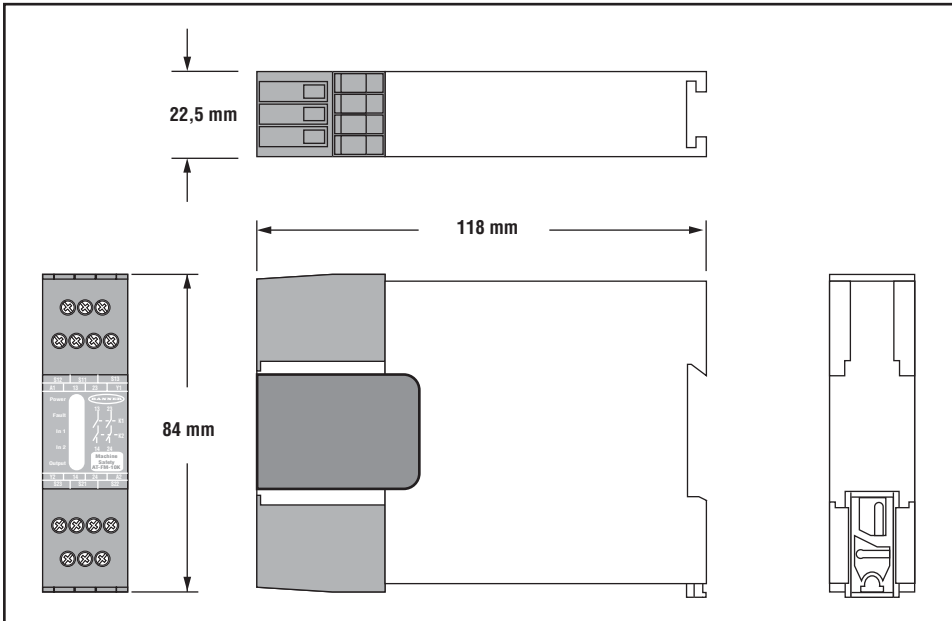
Figura 6. Dimensioni del modulo di sicurezza DUO-TOUCH SG
