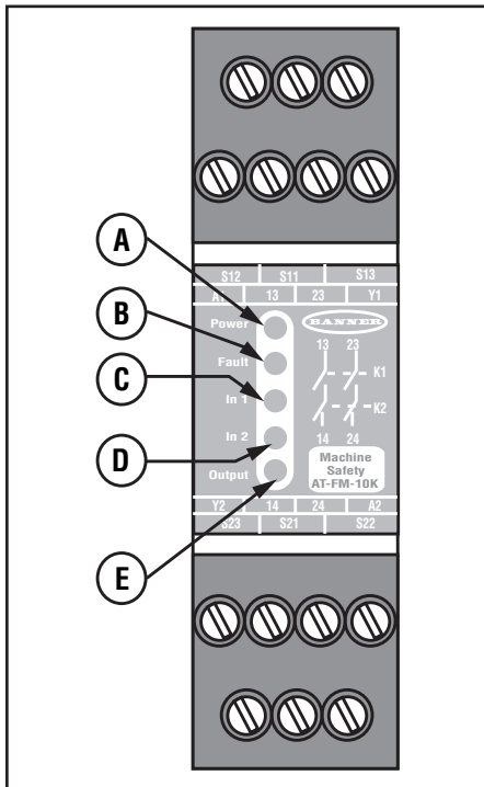
Figura 1. Modulo di sicurezza DUO-TOUCH SG AT-FM-10K – posizione degli indicatori di stato e dei morsetti
