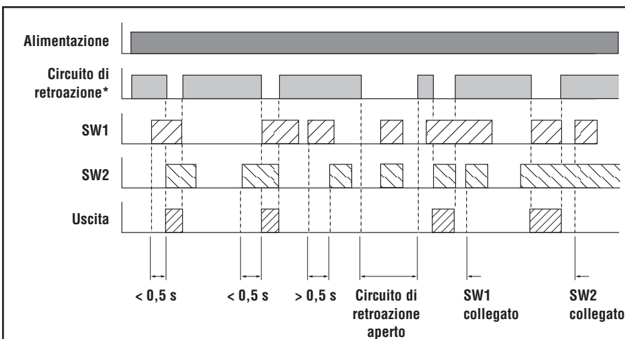
Figura 2. Diagramma temporale del modulo di sicurezza DUO-TOUCH SG AT-FM-10K
