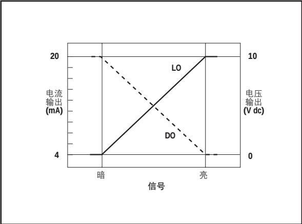
图2. 模拟量输出－双点示教（静态或动态）
