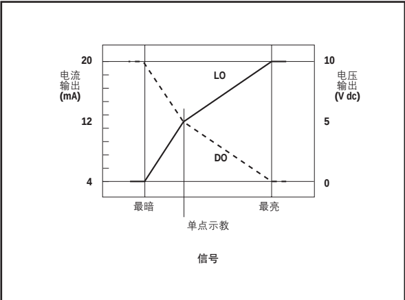
图3. 模拟量输出－单点示教
