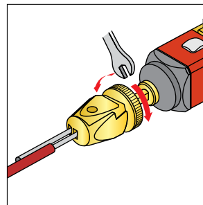
Figura 10. Applicazione di tensione alla fune (modelli RP-LS42F...LF)
