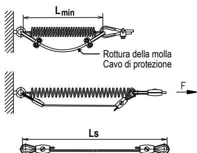
Figura 4. Molle di tensionamento singole
