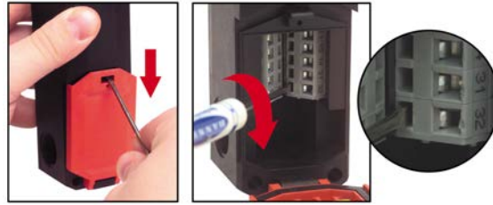
Figura 12. Accesso alla morsettiera
