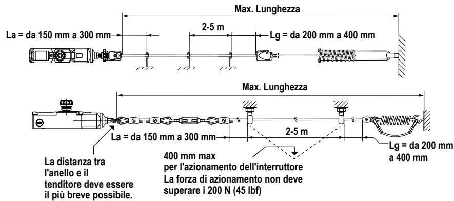
Figura 6. Montaggio della fune e della viteria
