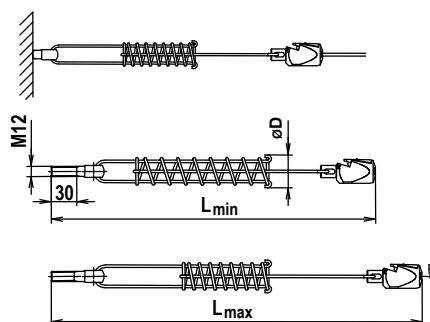
Figura 5. Gruppo molla di tensionamento
