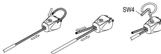
Figura 7. Installare la fune con il tenditore integrato
