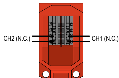
Figura 13. Contatti di sicurezza a 21/22 e 41/42
