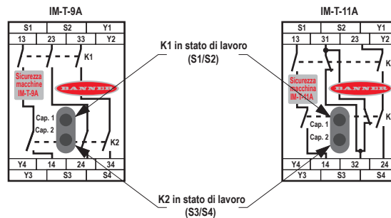
Figura 1. Indicatori di stato sul modulo di interfaccia
