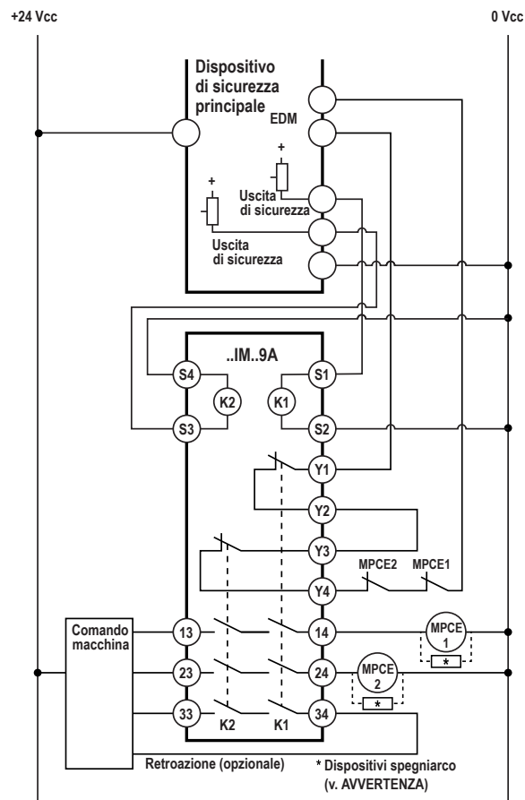
Figura 6. Esempio di collegamento a un dispositivo di sicurezza principale a 2 canali, con due uscite di sicurezza a corrente positiva e un ingresso di monitoraggio.
