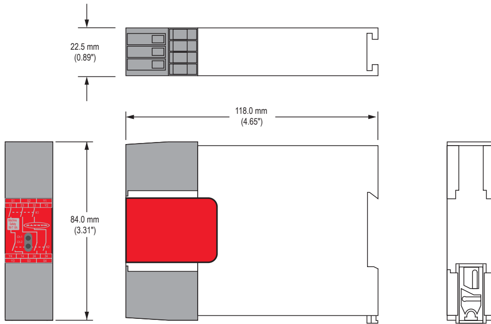
Figura 9. Dimensioni del modulo di interfaccia
