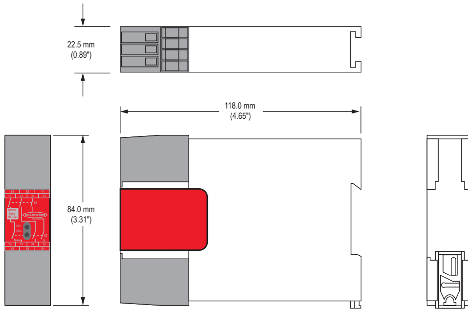
Illustration 9. Dimensions du module d'interface
