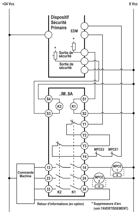
Illustration 6. Raccordement générique d'un dispositif primaire de sécurité à 2 voies avec deux sorties de sécurité en intensité et une entrée de surveillance.
