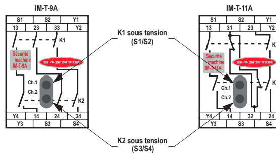
Illustration 1. LED d'état du module d'interface
