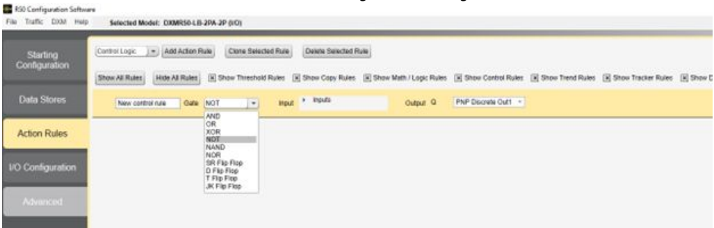
Schermata delle regole Control Logic
