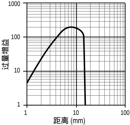
图4. 过量增益 (15 毫米型号)
