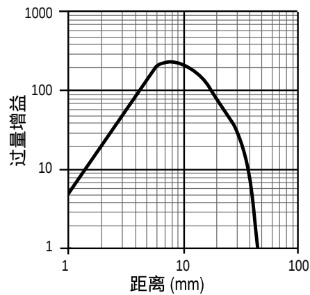
图6. 过量增益 (45 毫米型号)
