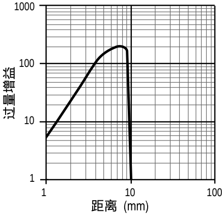
图3. 过量增益 (10 毫米型号)
