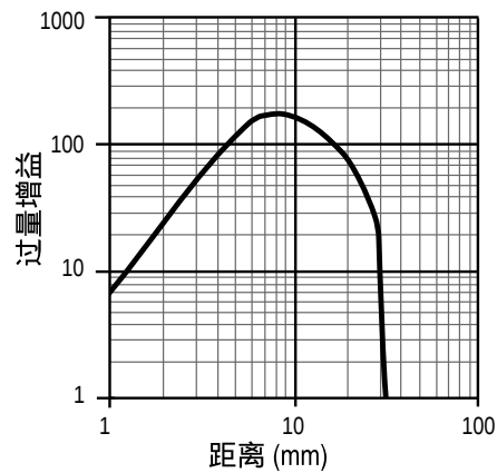
图5. 过量增益 (30 毫米型号)
