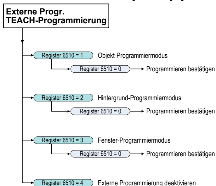
Übersicht über den externen Programmieingang
