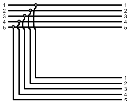
Inline-Ausführungen
