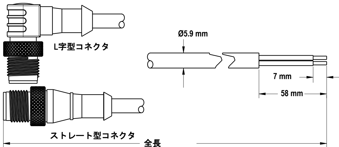
図 1: ワイヤ寸法
