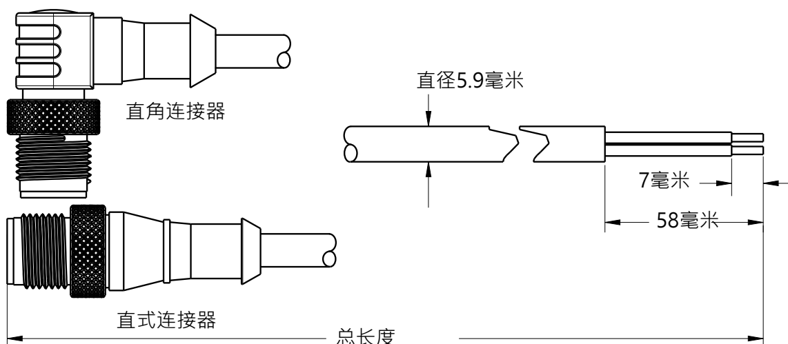
图 1: 电线尺寸
