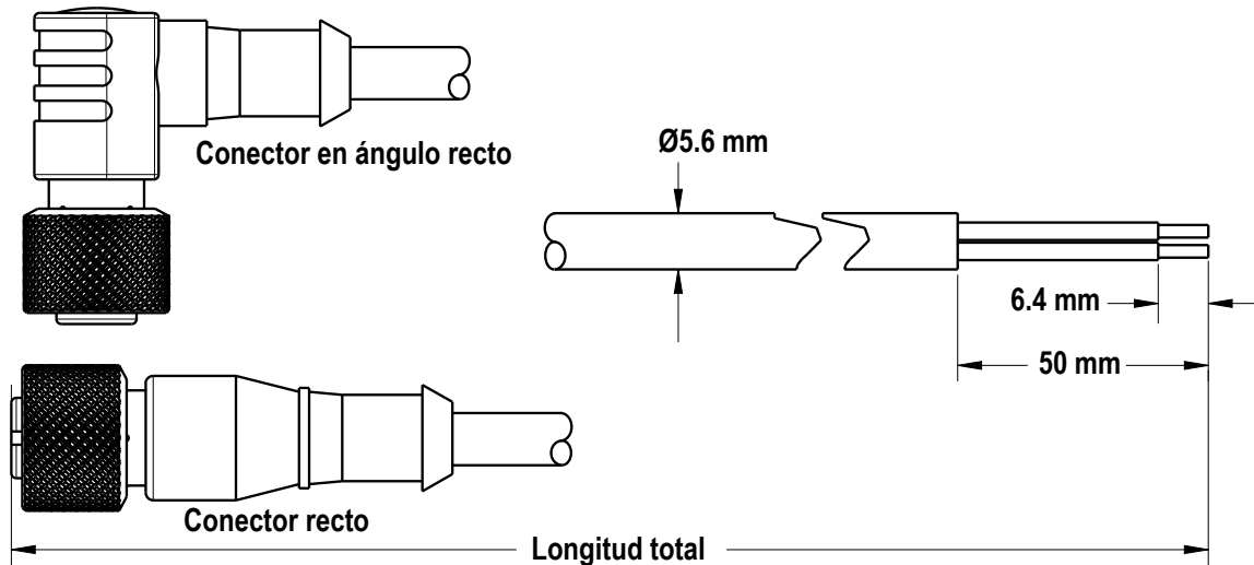
Imagen 1: Dimensiones del cable
