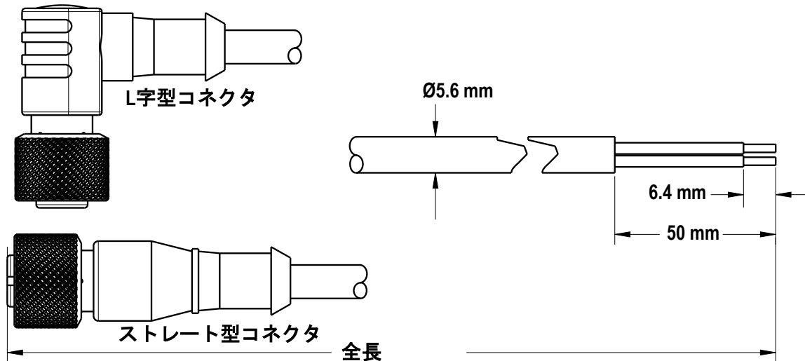
図 1: ワイヤ寸法
