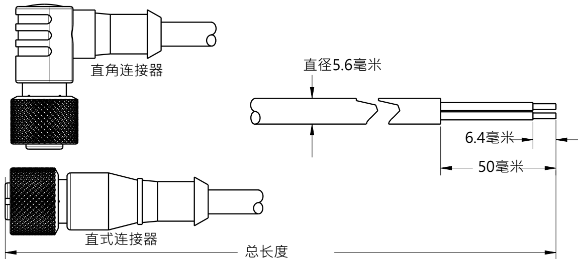
图 1: 电线尺寸
