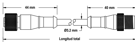
Imagen 5: Dimensiones de MQDEC..RS
