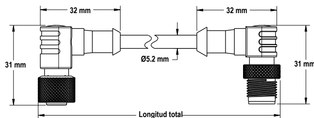
Imagen 6: Dimensiones de MQDEC..RR
