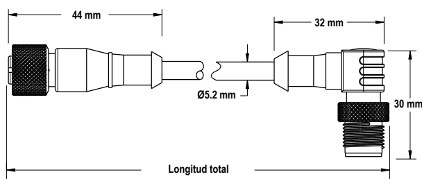
Imagen 6: Dimensiones de MQDEC..RR
