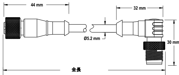
図 6: MQDEC..RR 寸法
