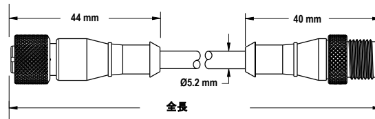
図 5: MQDEC..RS 寸法
