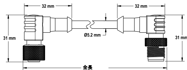
図 6: MQDEC..RR 寸法
