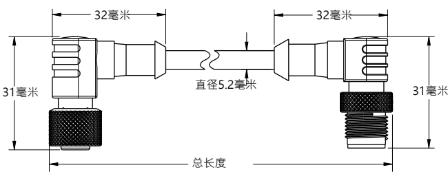
图 6: MQDEC.RR 尺寸
