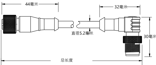
图 6: MQDEC.RR 尺寸
