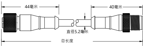
图 5: MQDEC.RS 尺寸
