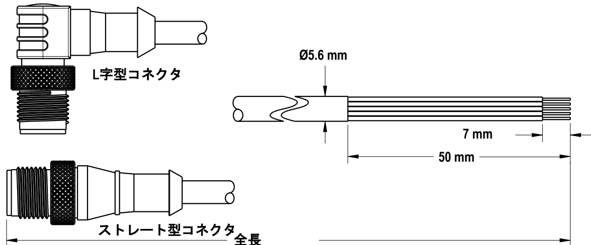
図 1: ワイヤ寸法
