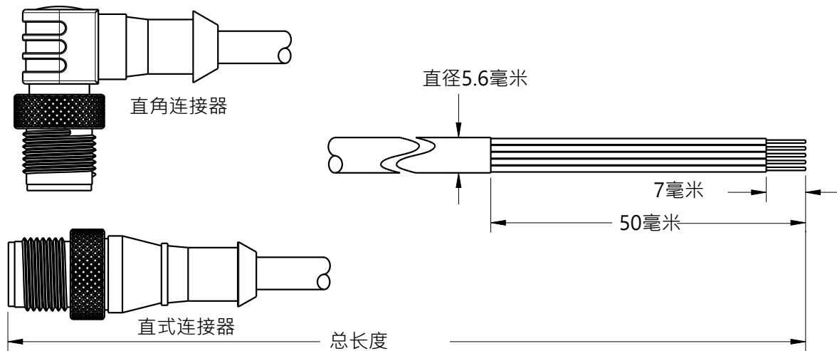
图 1: 电线尺寸
