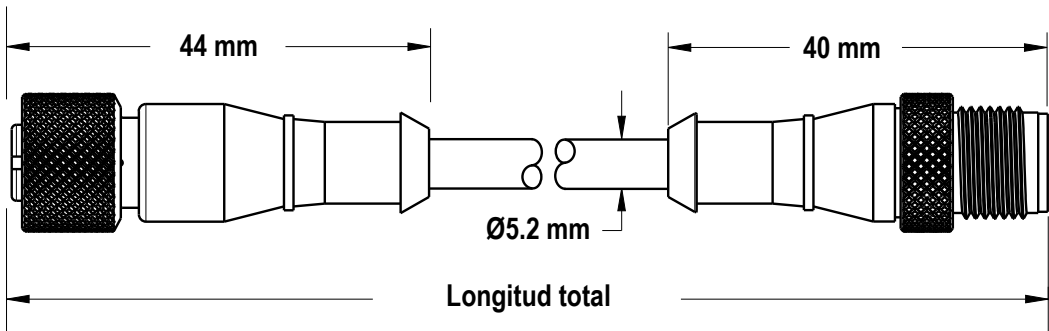
Imagen 1: Dimensiones del cable
