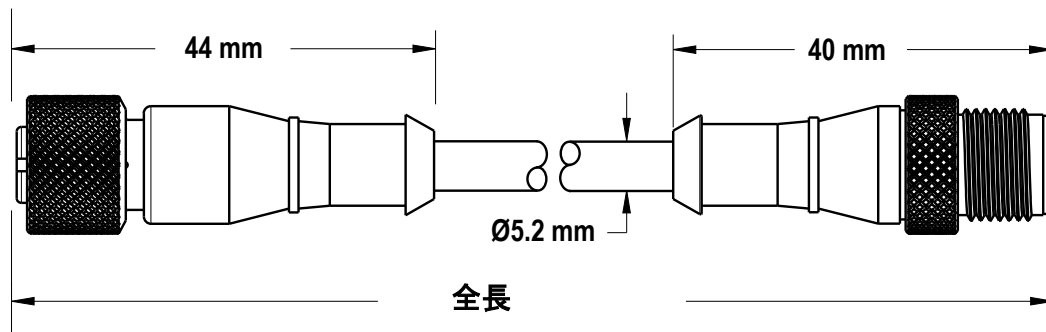
図 1: ワイヤ寸法
