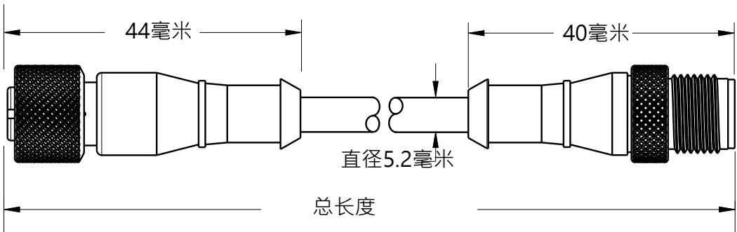
图 1: 电线尺寸
