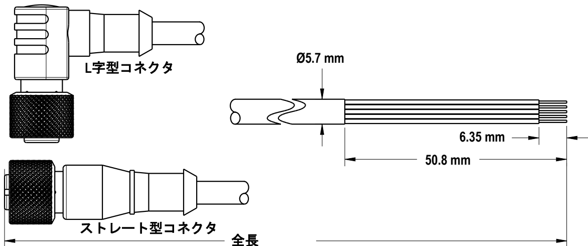
図 1: ワイヤ寸法
