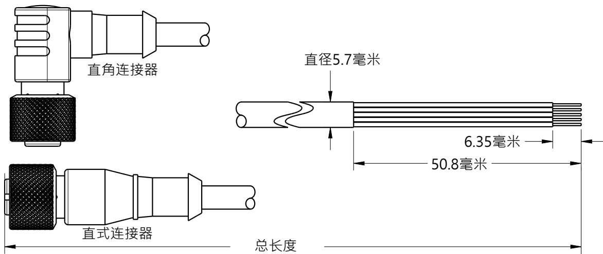
图 1: 电线尺寸
