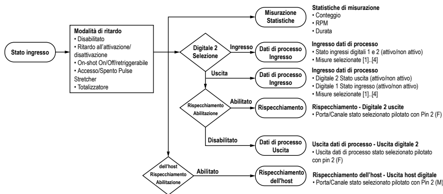
Figura 1. Flusso logico
