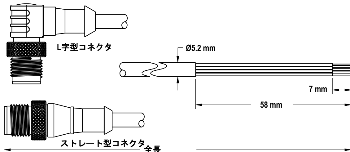
図 1: ワイヤ寸法
