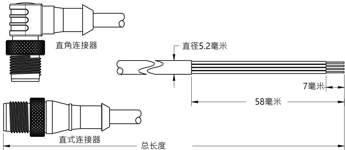
图 1: 电线尺寸
