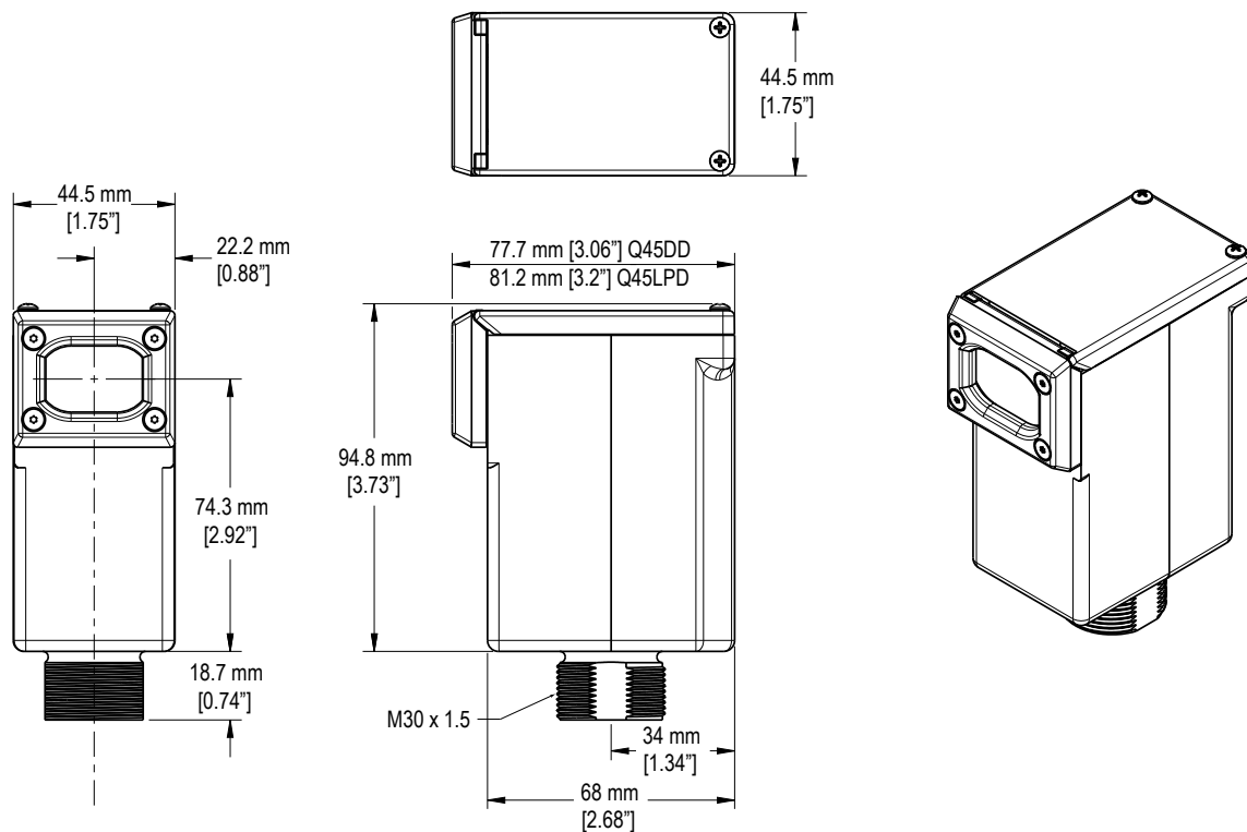
Q45UPSD Dimensions
