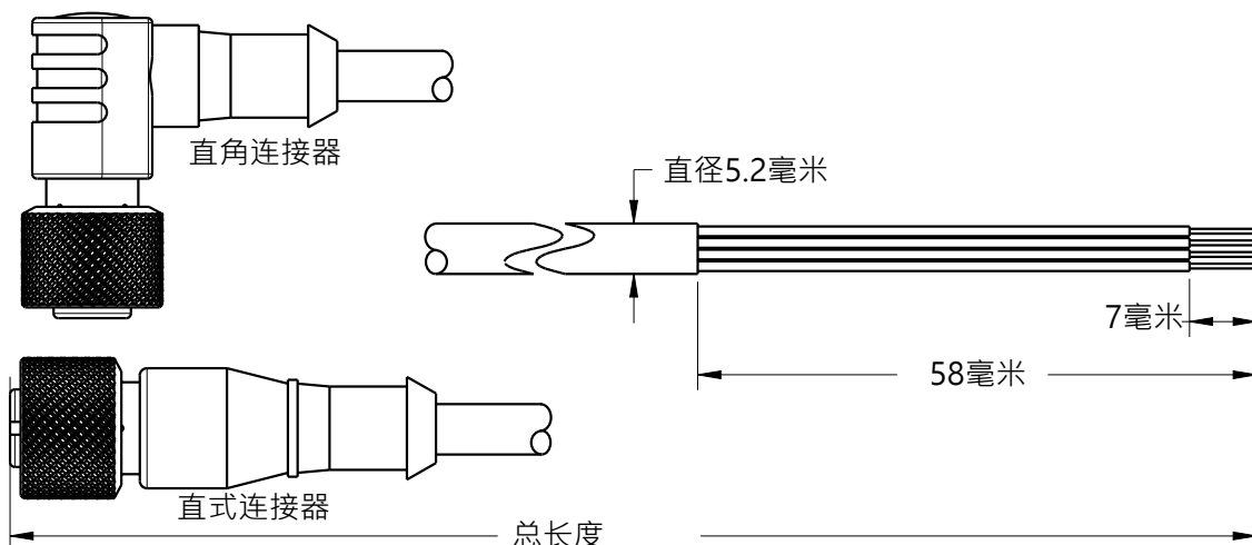
图 1: 电线尺寸
