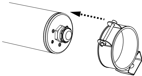
Figura 1. Fissaggio delle staffe di serraggio (punto 3)
