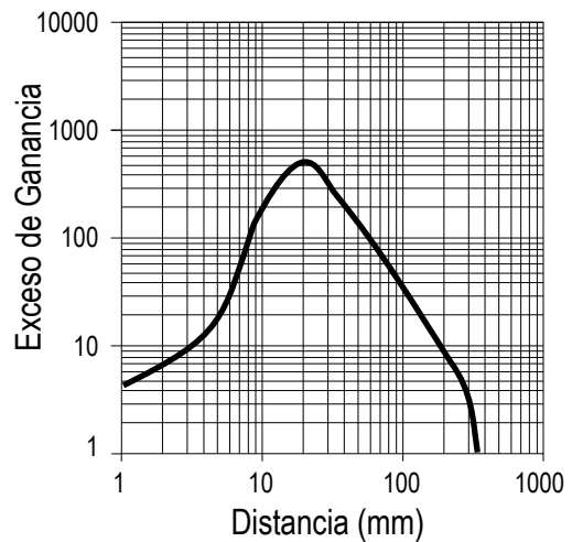
Curva de exceso de ganancia con corte de 350 mm (según la tarjeta blanca al 90 %)
