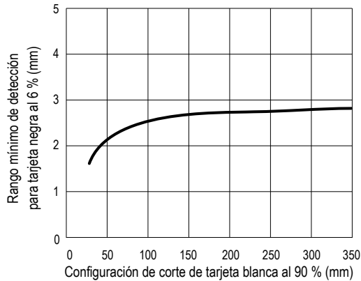
Rango mínimo de detección (zona muerta) en función de la configuración de corte del blanco al 90 %
