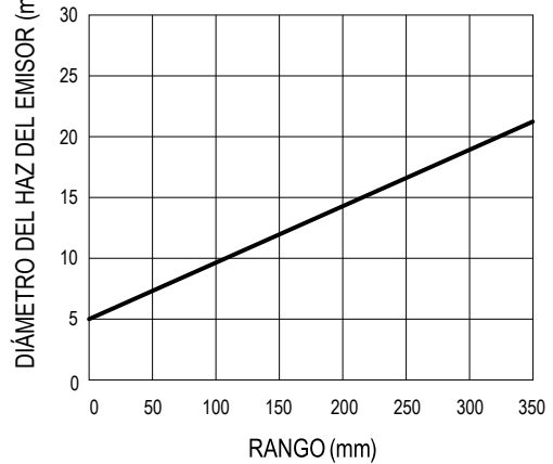
Diámetro típico del punto del emisor en función de la distancia
