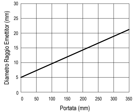
Diametro tipico dello spot dell'emettitore vs. distanza
