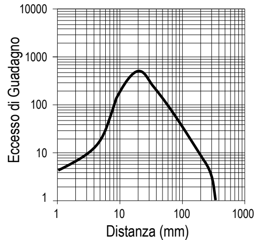
Curva dell'eccesso di guadagno con cutoff a 350 mm (utilizzando una carta bianca con riflettanza del 90%)
