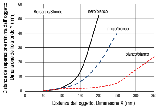
Distanza minima di separazione tra l'oggetto e lo sfondo: modalità di soppressione dello sfondo
