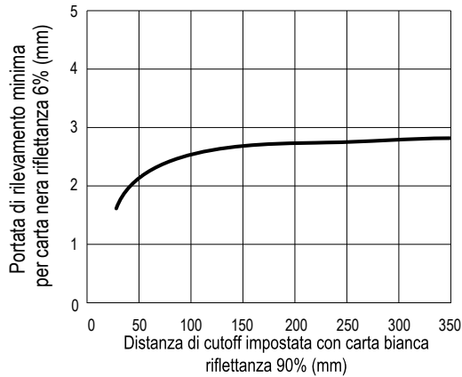
Distanza di rilevamento minima (zona morta) vs. distanza di cutoff impostata con carta bianca a riflettanza 90%
