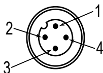
M12 mâle à 4 broches
