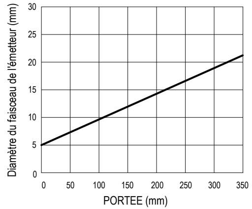
Diamètre typique du faisceau de l'émetteur en fonction de la distance
