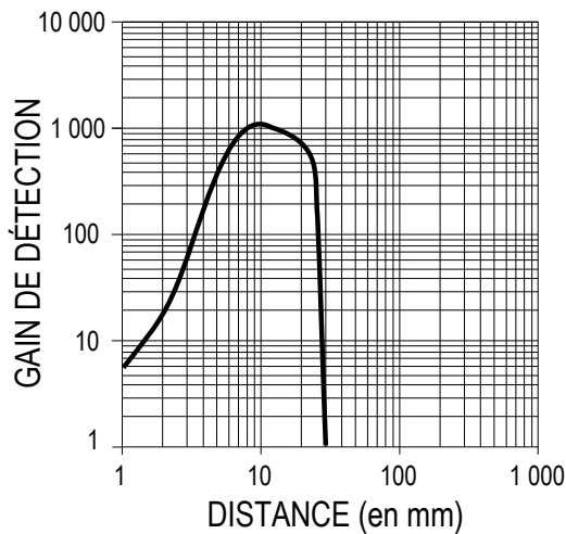
Courbe de gain de détection avec limite du seuil de détection à 30 mm (basée sur une carte blanche 90%)
