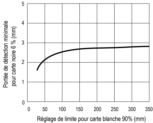
Portée minimale de détection (zone morte) par rapport à la configuration de la distance limite avec une cible à 90 % blanc
