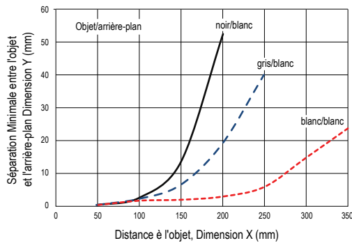
Distance de séparation minimale entre l'objet et l'arrière-plan : mode à suppression d'arrière-plan
