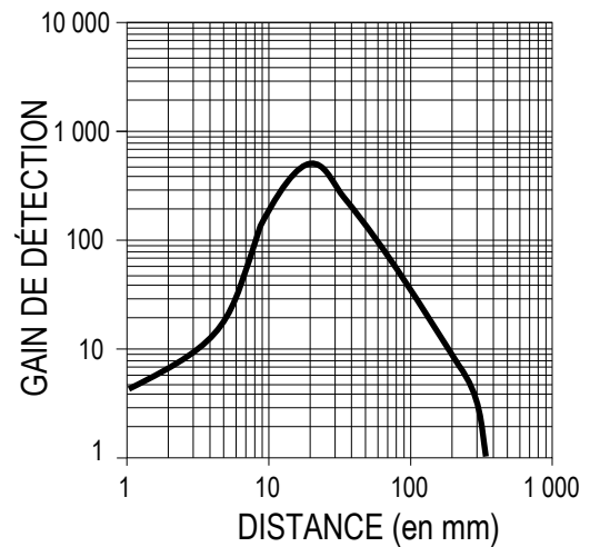
Courbe de gain de détection avec limite du seuil de détection à 350 mm (basée sur une carte blanche 90%)
