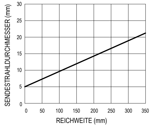
Typischer Sender-Lichtpunktdurchmesser in Relation zur Reichweite
