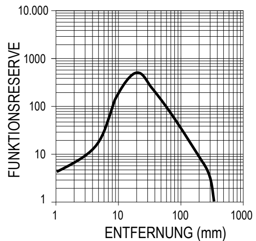
Funktionsreservekurve mit 350 mm Ausblendgrenze (bei weißer Karte mit 90% Reflexionsvermögen)
