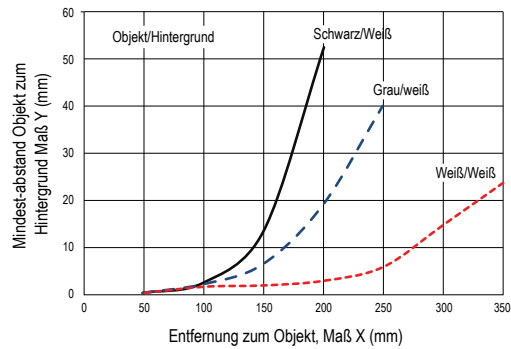
Mindestabstand zwischen Objekt und Hintergrund: Hintergrundausbldung
