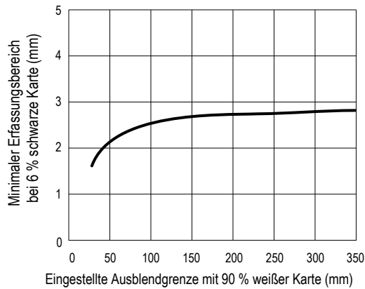
Mindestreichweite (Totbereich) in Relation zur eingestellten Ausblendgrenze mit 90% weißer Karte
