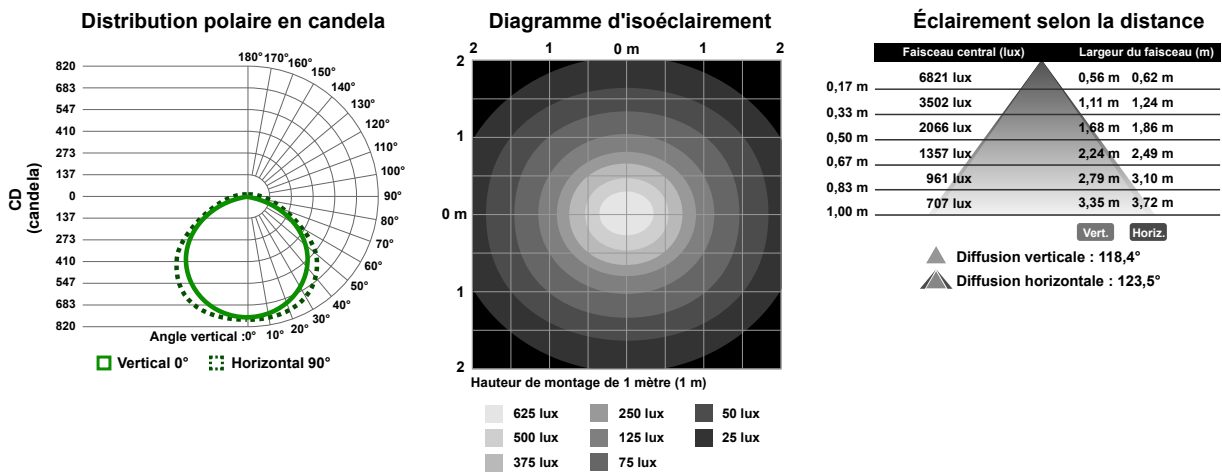
Illustration 10. Modèles 1130 mm
