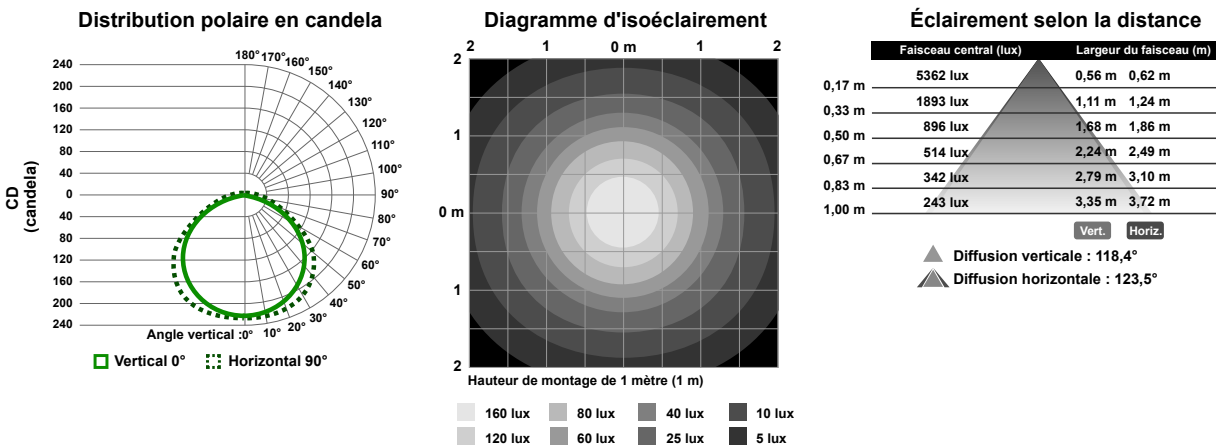
Illustration 4. Modèles 285 mm
