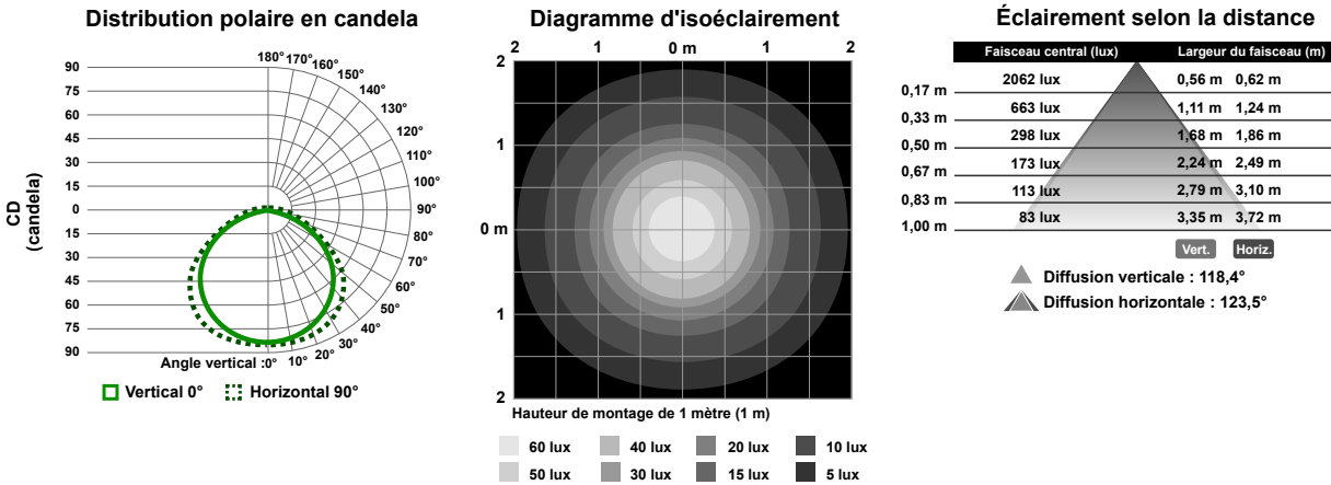
Illustration 4. Modèles 285 mm
