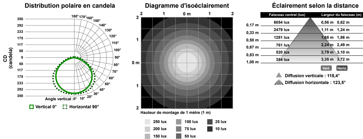
Illustration 6. Modèles 570 mm
