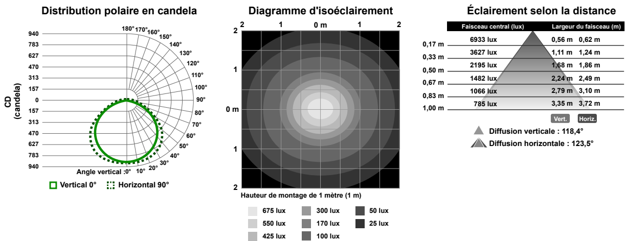
Illustration 10. Modèles 1130 mm
