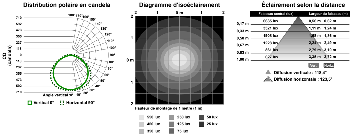
Illustration 9. Modèles 990 mm
