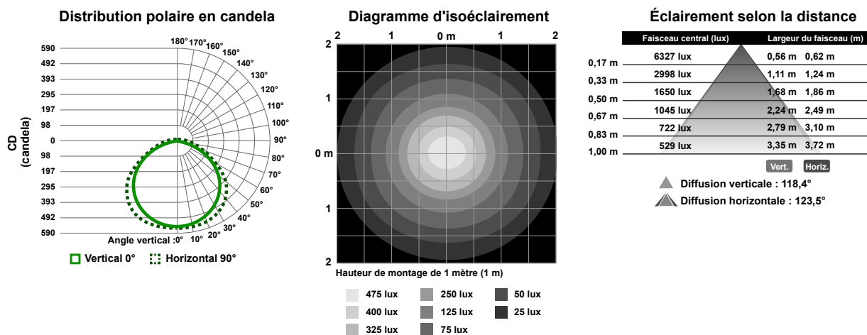
Illustration 7. Modèles 710 mm
