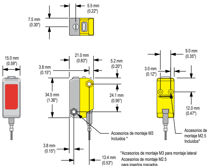
Dimensiones de QS18CV20
