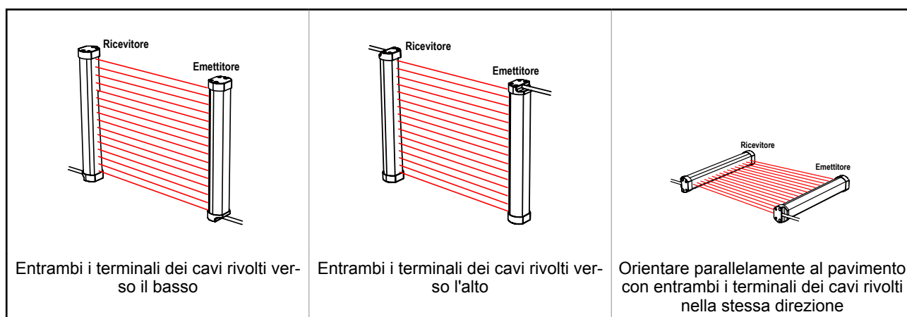
Figura 6. Esempi di orientamento corretto dell'emettitore e ricevitore
