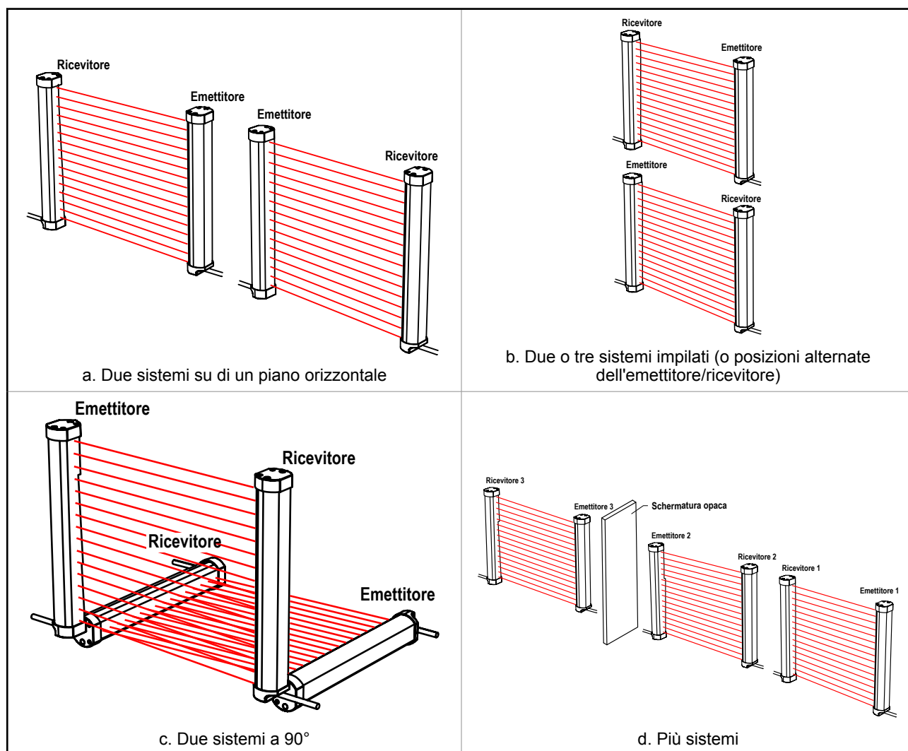
Figura 8. Installazione di più sistemi
