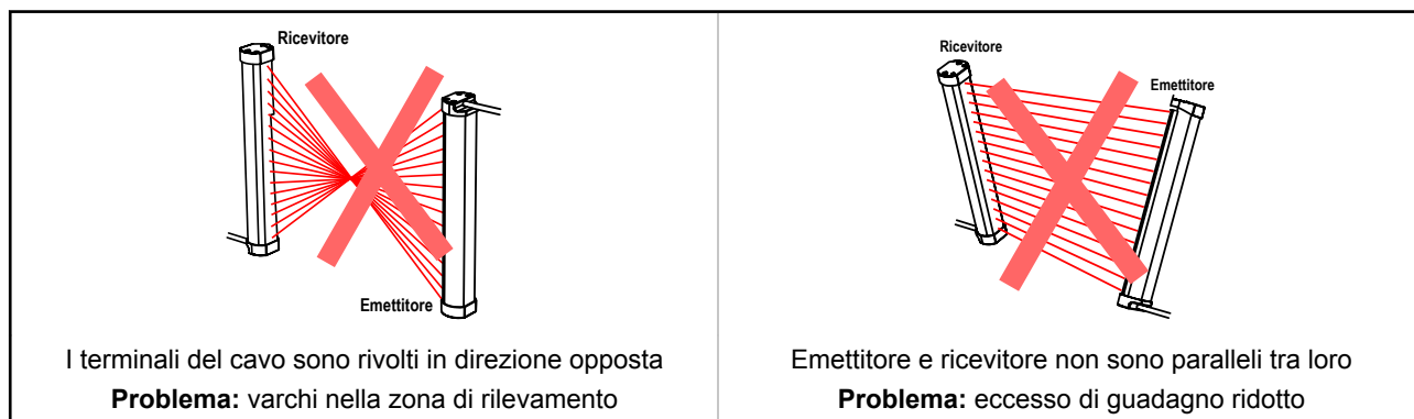
Figura 7. Esempi di orientamento non corretto dell'emettitore e del ricevitore
