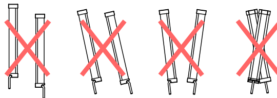
Figura 13. Allineamento sensore non corretto
