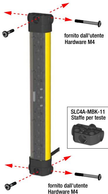
Figura 9. Staffe per montaggio tramite testa
