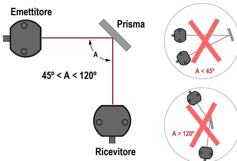
Figura 5. Utilizzo dei sensori SLC4 in modalità a riflessione
