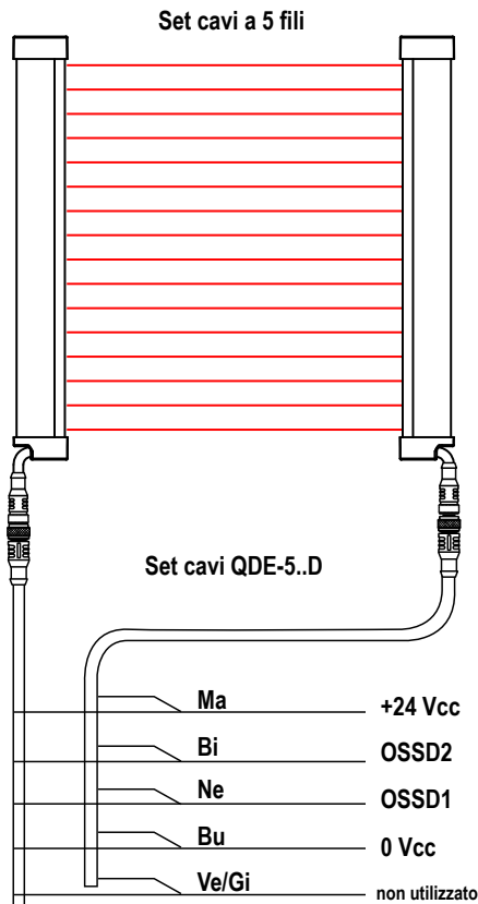
Figura 15. Set cavi singoli
