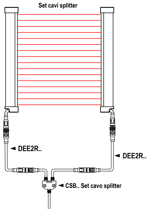
Figura 16. Set cavi splitter
