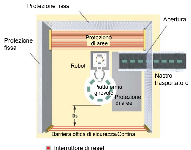
Figura 3. Un esempio di protezione supplementare
