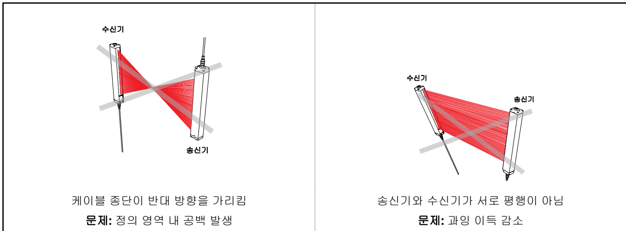
그림 13: 부정확한 송신기/수신기 방향의 예
