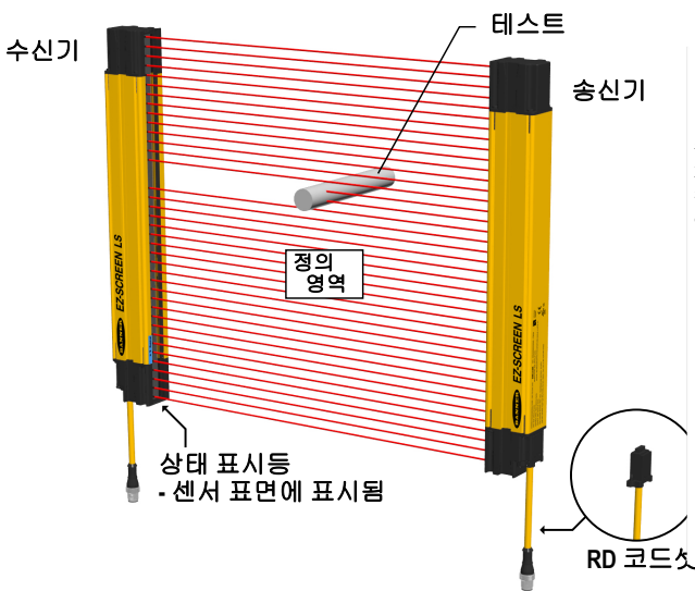
그림 1: EZ-SCREEN LS Basic 시스템: 송신기, 수신기, 상호 연결 코드셋
