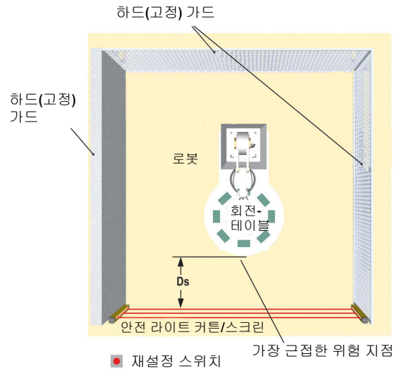
그림 8: 안전 거리(최소 거리) 및 하드(고정) 가드
