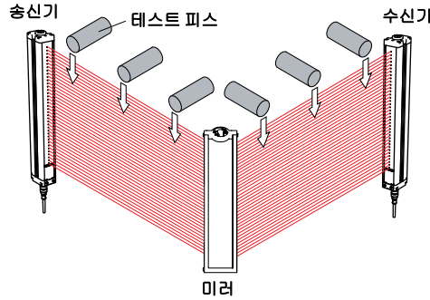
그림 25: 코너 미러를 사용한 트립 테스트
