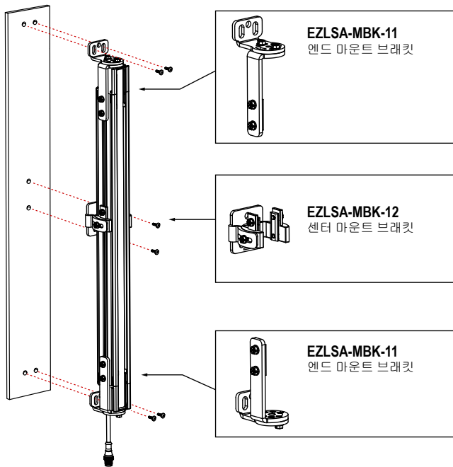
그림 16: 센터 및 측면 마운트 브래킷 장착
