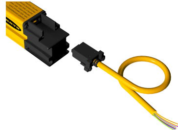
그림 4: 8와이어 플라잉 리드 코드셋을 사용한 RD 연결
