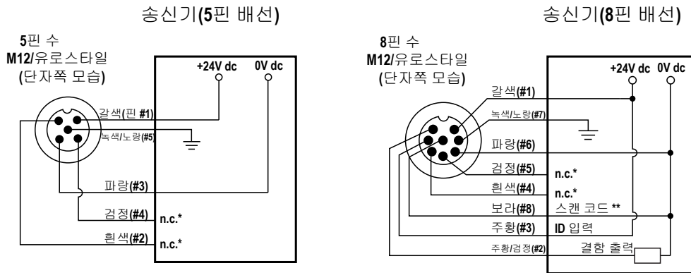
그림 29: 일반 배선도 - 송신기
