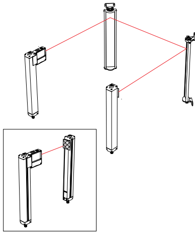
그림 22: LAT-1-SS를 사용한 광학 정렬
