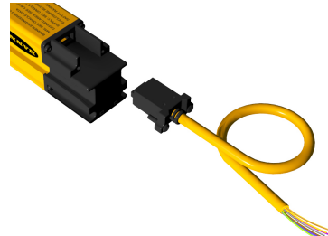
그림 36: 8와이어 플라이 리드 코드셋을 사용한 RD 연결
