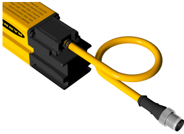
그림 3: 300 mm 피그테일 + M12/유로스타일 QD
