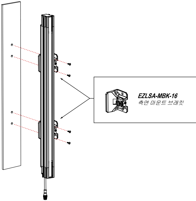
그림 17: 측면 마운트 브래킷
