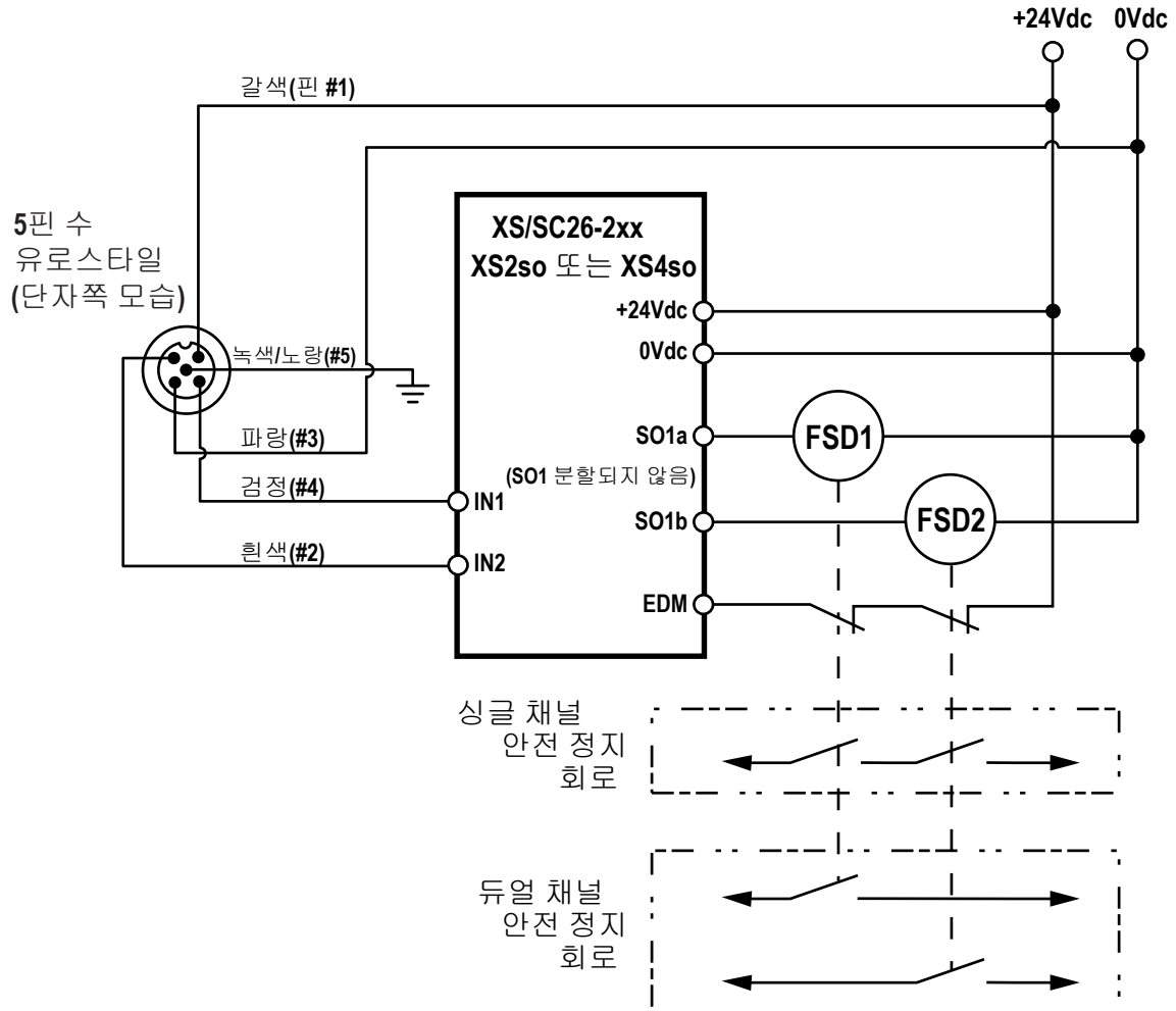
그림 32: 일반 배선도 - XS/SC26-2 안전 컨트롤러
