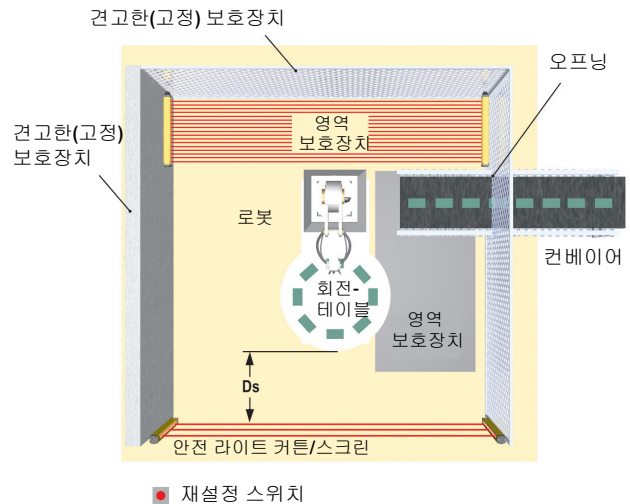
그림 9: 보조 안전장치의 예
