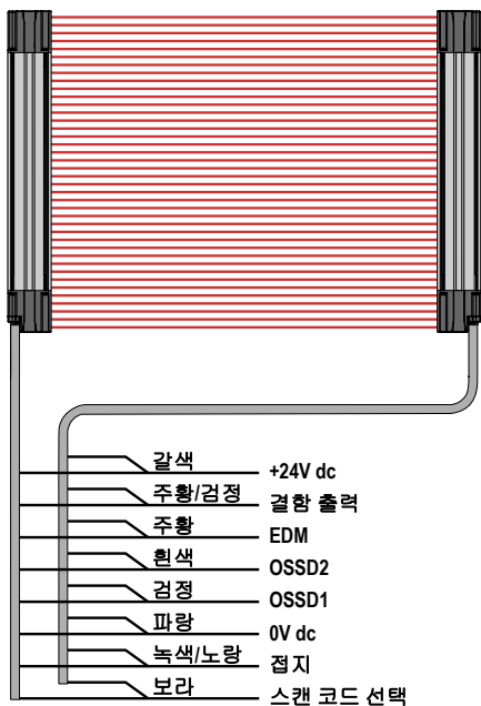
그림 27: 개별 코드셋
