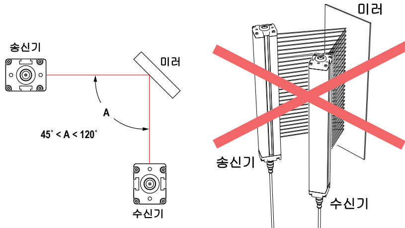
그림 11: 재귀반사 모드에서 EZ-SCREEN LS Basic 센서 사용
