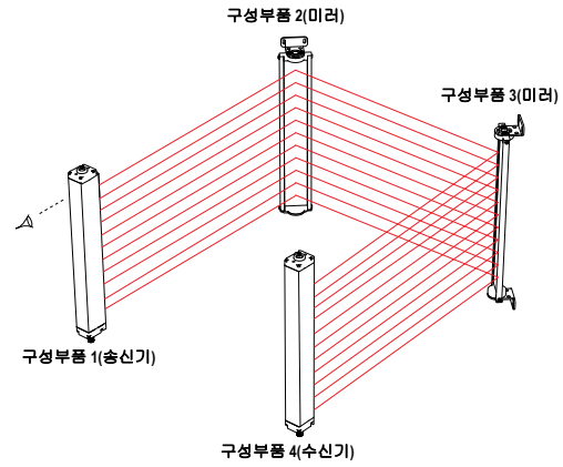
그림 23: 코너 미러 정렬
