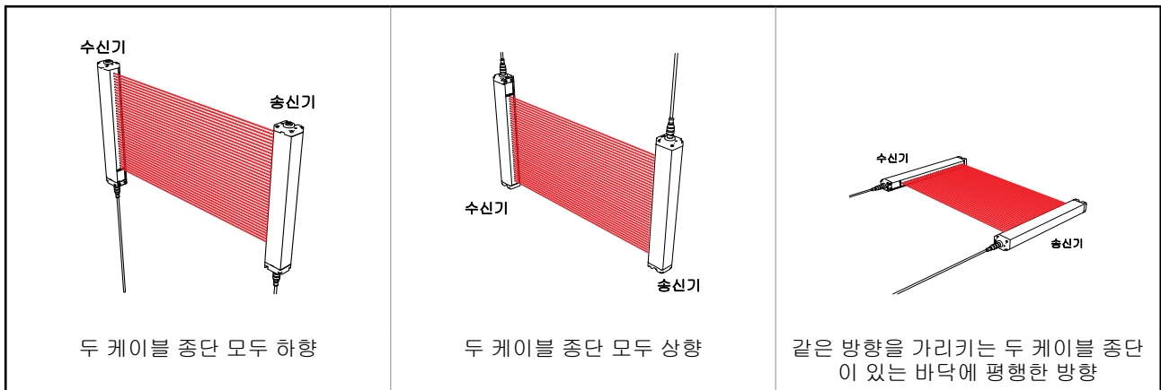
그림 12: 정확한 송신기/수신기 방향의 예
