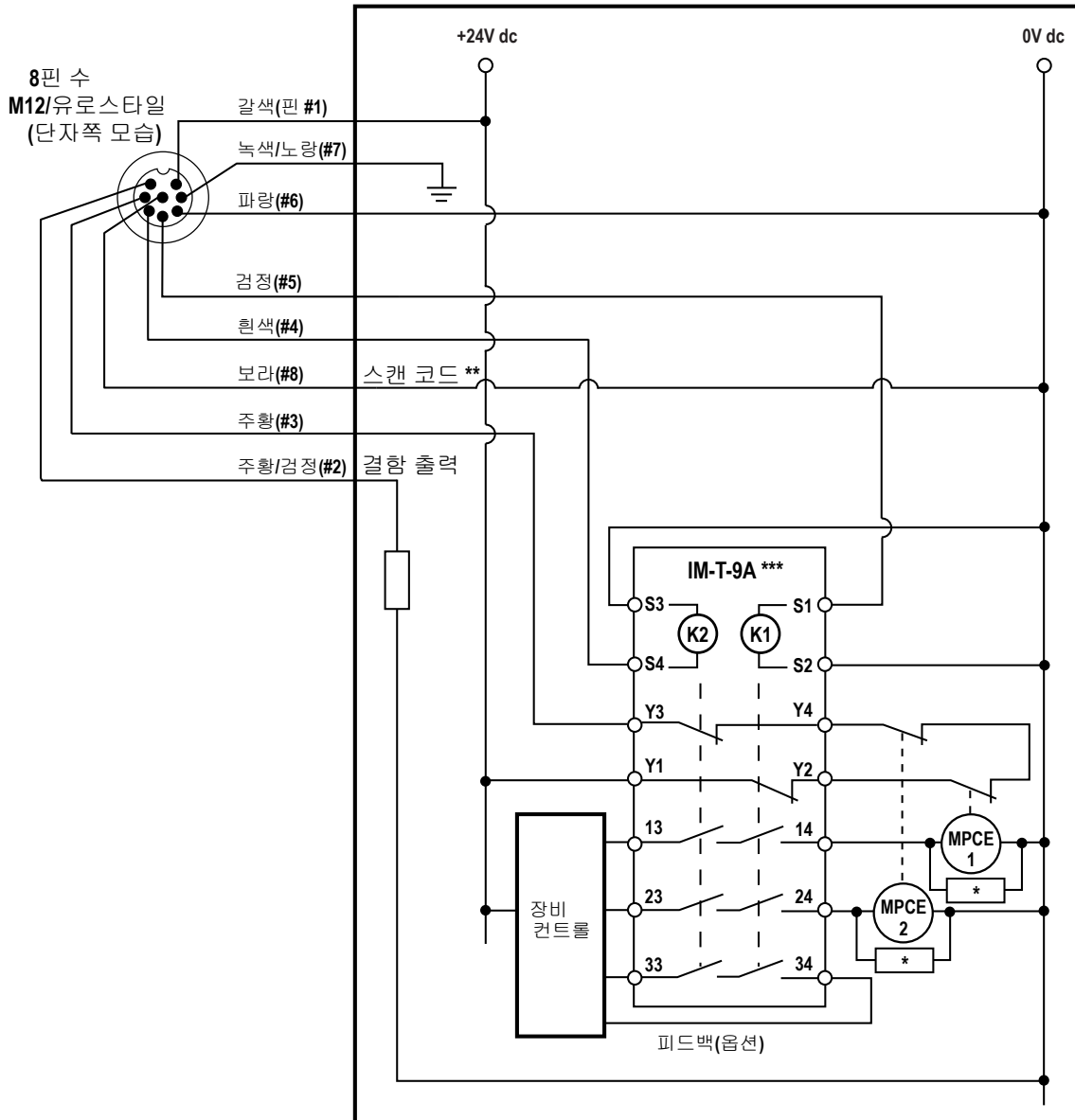
그림 34: 일반 배선도 - IM-T-9A 인터페이스 모듈(1채널 EDM)
