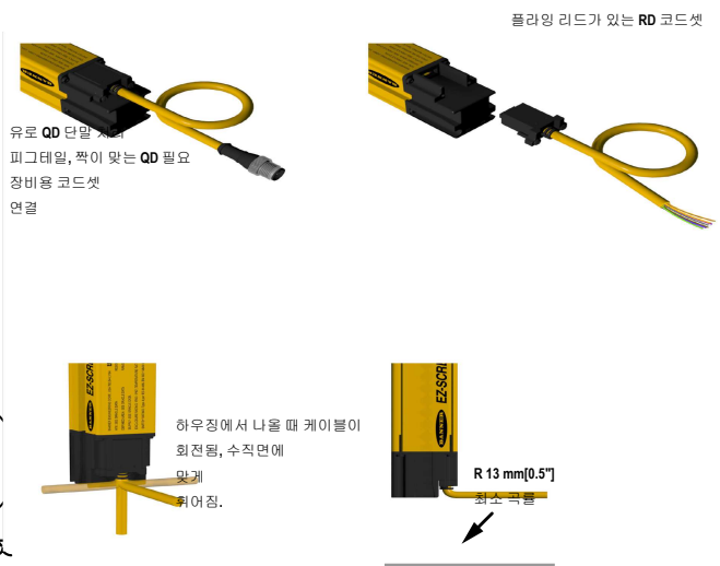
그림 2: EZ-SCREEN LS Basic 코드셋 옵션
