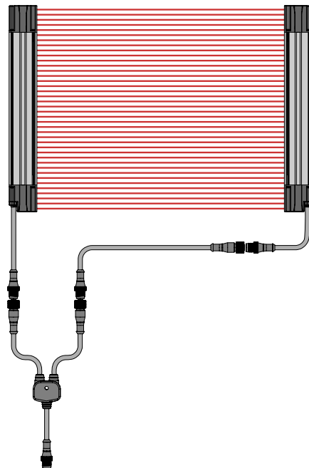
그림 28: 스플리터 코드셋
