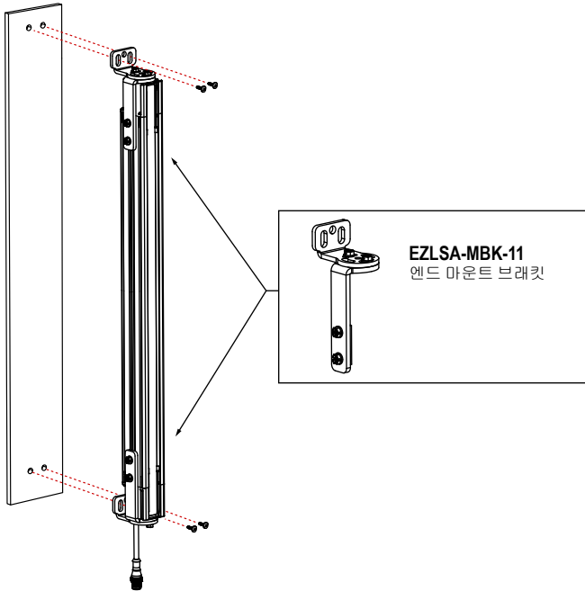
그림 15: 엔드 마운트 브래킷
