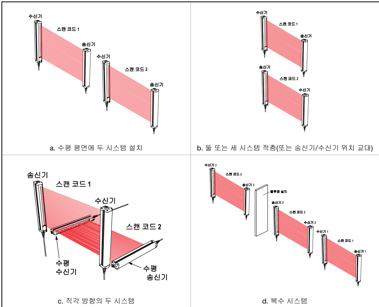
그림 14: 복수 시스템 설치
