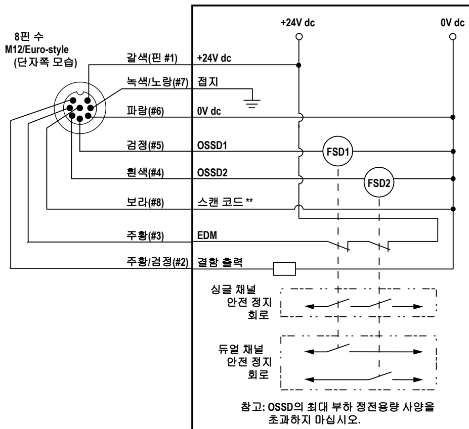
그림 33: 일반 배선도 - 8핀 수신기 및 이중화 FSD
