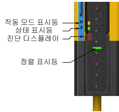
그림 7: 상태 표시등 - 수신기
