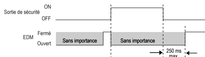
Illustration 27. État de l'EDM à une voie par rapport à la sortie de sécurité
