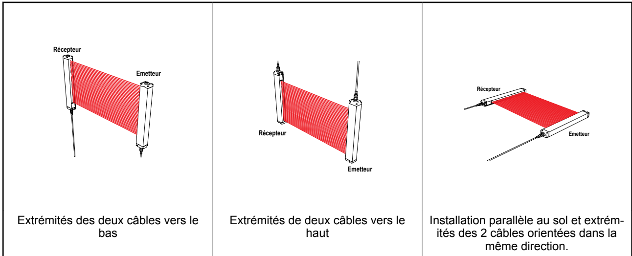
Illustration 16. Exemples d'orientation correcte de l'émetteur et du récepteur
