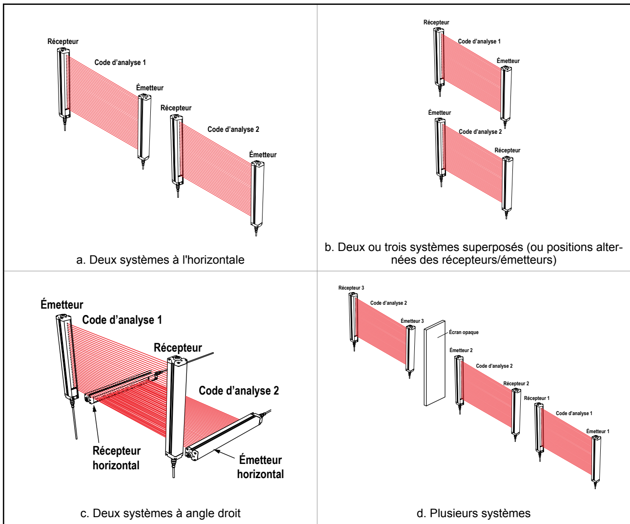
Illustration 18. Installation de plusieurs systèmes
