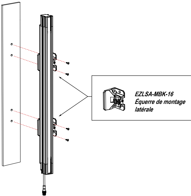
Illustration 21. Équerre de montage latéral
