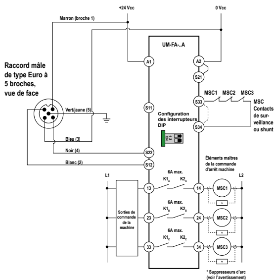
Illustration 31. Schéma de câblage générique - Module UM-FA..A avec reset automatique
