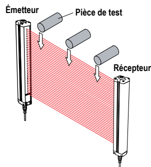
Illustration 25. Test de fonctionnement
