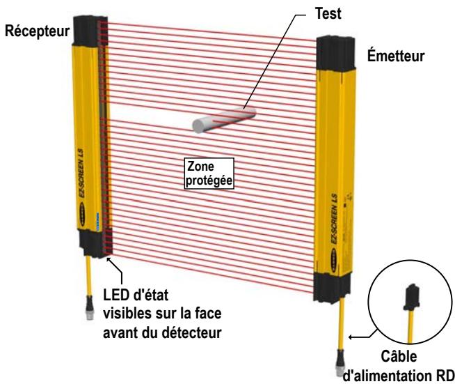
Illustration 1. Système EZ-SCREEN LS Basic : émetteur, récepteur et câbles de raccordement
