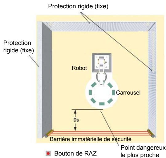
Illustration 12. Distance de sécurité (minimale) et protection fixe
