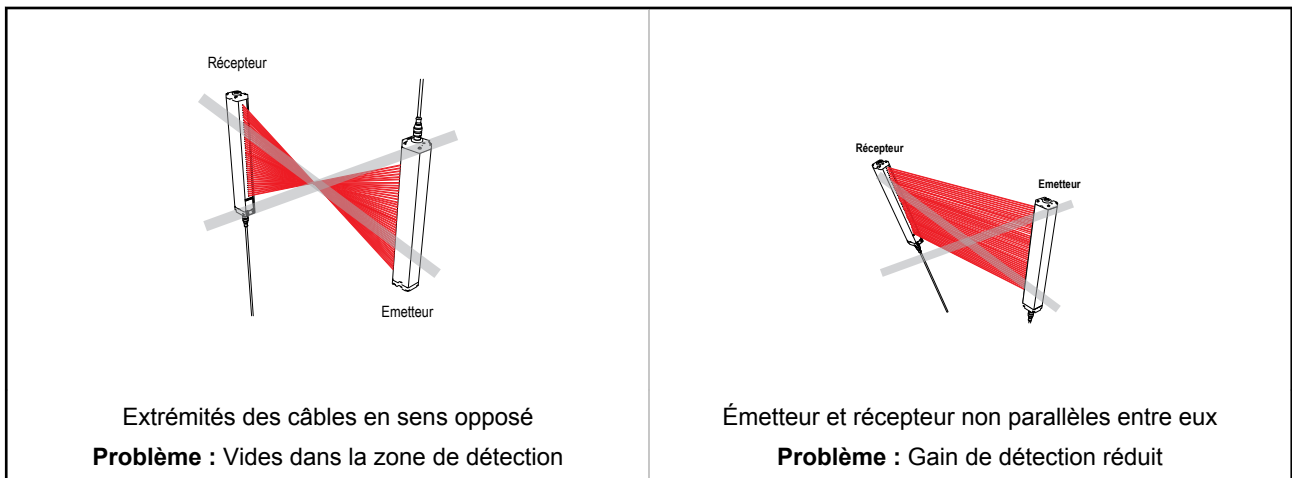
Illustration 17. Exemples d'orientation incorrecte de l'émetteur et du récepteur
