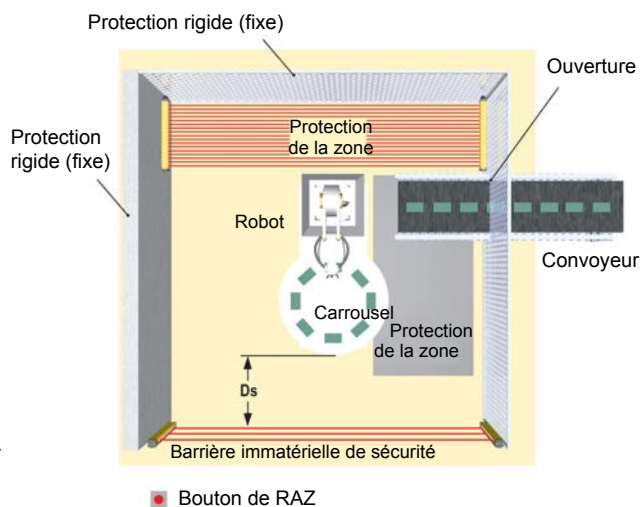
Illustration 13. Exemple de protection supplémentaire
