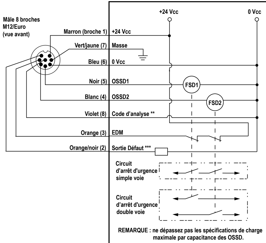
Illustration 34. Schéma de câblage générique — Récepteur à 8 broches et dispositifs de commutation finaux redondants (FSD)
