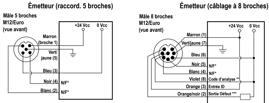
Illustration 30. Schéma de câblage générique — Émetteur
