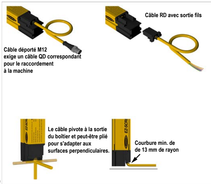
Illustration 2. Options de raccordement du système EZ-SCREEN LS Basic
