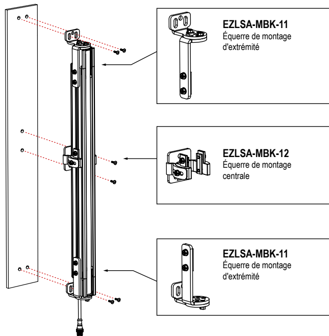
Illustration 20. Montage des équerres centrales et latérales
