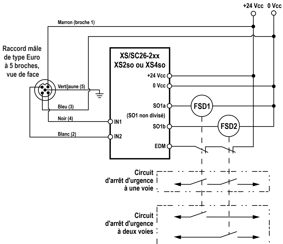
Illustration 33. Schéma de câblage générique — Contrôleur de sécurité XS/SC26-2
