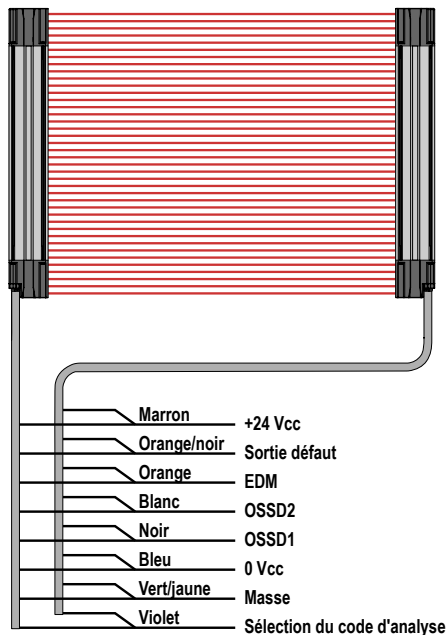
Illustration 28. Câbles individuels
