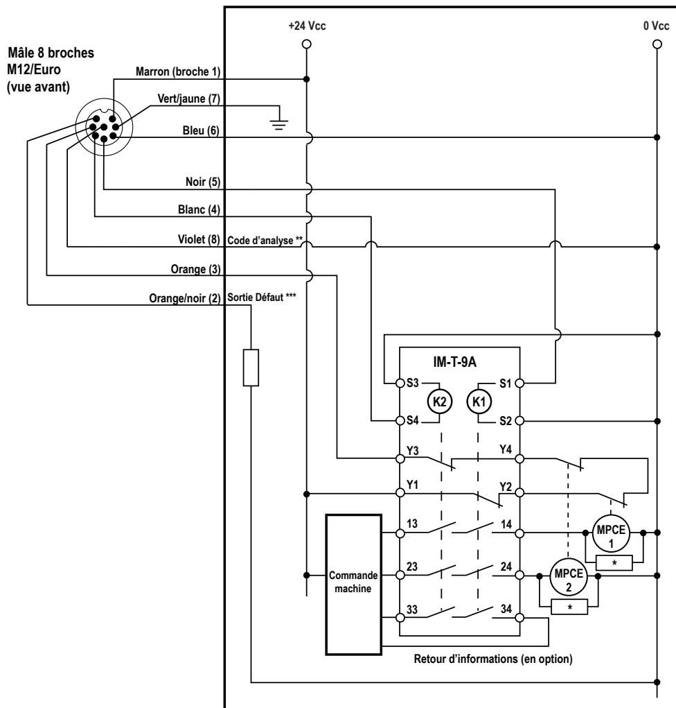
Illustration 35. Schéma de câblage générique — Module d'interface IM-T-9A (EDM simple voie)
