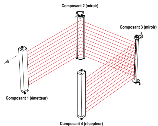
Illustration 24. Alignement des miroirs d'angle
