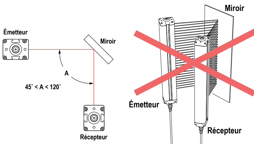
Illustration 15. Utilisation des capteurs EZ-SCREEN LS Basic en mode rétro-réfléctif
