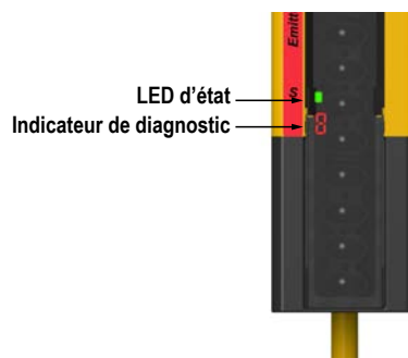
Illustration 6. LED d'état — Émetteur
