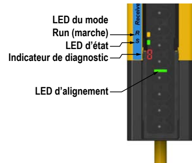
Illustration 7. LED d'état — Récepteur
