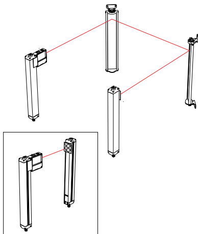
Illustration 23. Alignement optique à l'aide de l'outil LAT-1-SS
