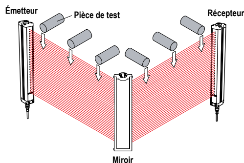
Illustration 26. Test de fonctionnement avec miroir d'angle
