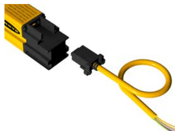
Illustration 4. Câble avec sortie 8 fils
