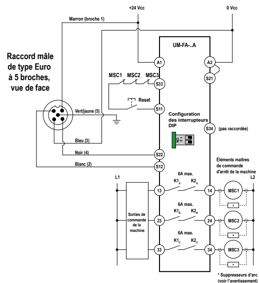
Illustration 32. Schéma de câblage générique - Module UM-FA..A avec reset manuel
