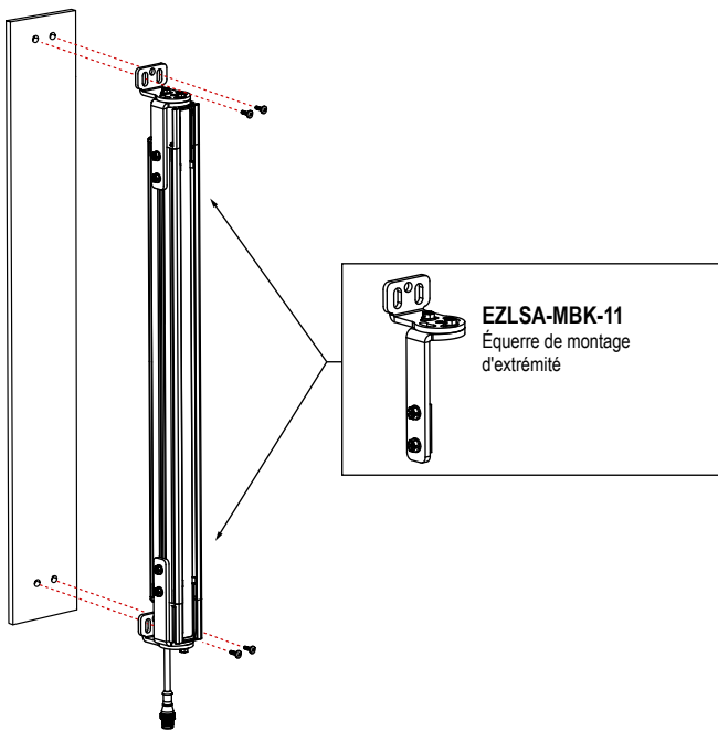
Illustration 19. Équerres d'extrémité
