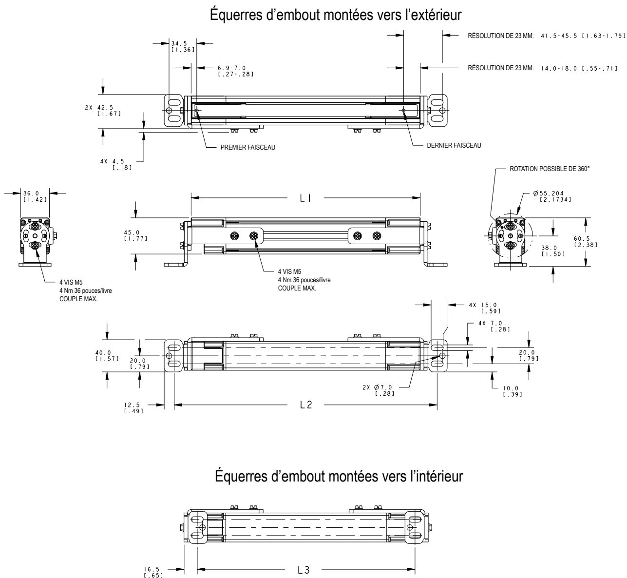
Illustration 8. Dimensions indiquées avec l'équerre EZLSA-MBK-11
