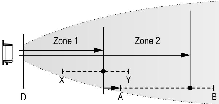
R-GAGE 设定点距离
